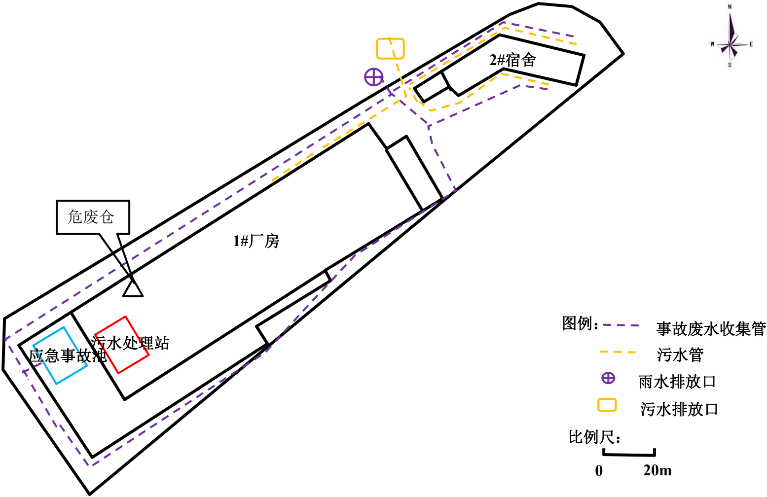
图 5-53 项目事故废水收集管道布置图
