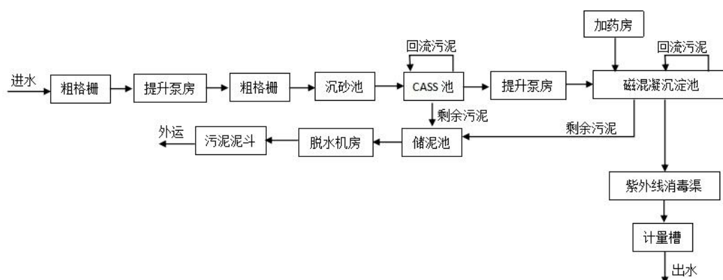
图 5-46 中山市港口污水处理有限公司污水处理工艺图
