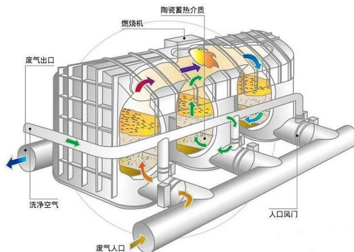
图 6-7 RTO 示意图
