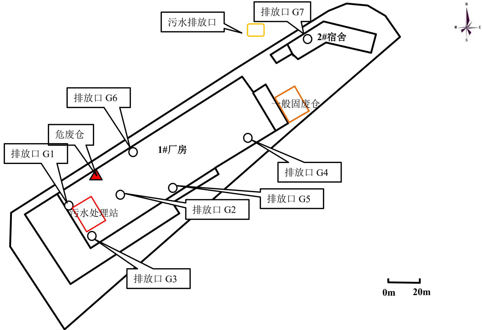
图 3-3 项目全厂平面布置图
