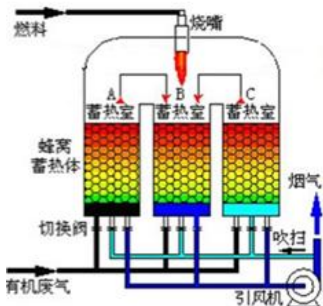
图 6-6 RTO 流程示意图
