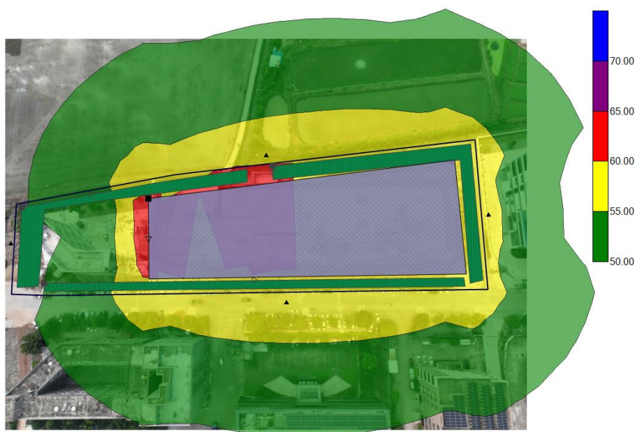
图 5-48 项目建成后噪声贡献等值线图
