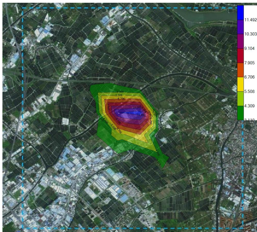
图 5-25 TSP 新增污染源最大日均质量浓度分布图
