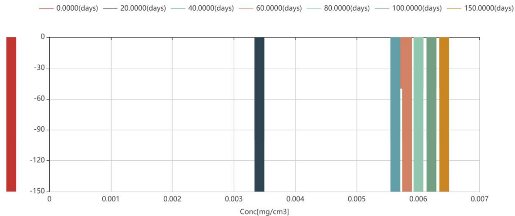
图 5-51 石油烃（C 10 -C 40 ）垂直入渗结果（深度变化）
