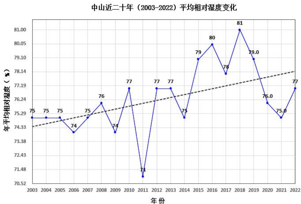
图 4-7 中山气象站年平均相对湿度变化（统计年限：2003-2022 年）
