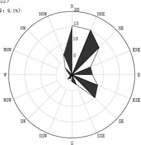
中山近二十年累年11月风向频率
