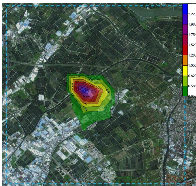
图 5-26 TSP 新增污染源最大年平均质量浓度分布图
