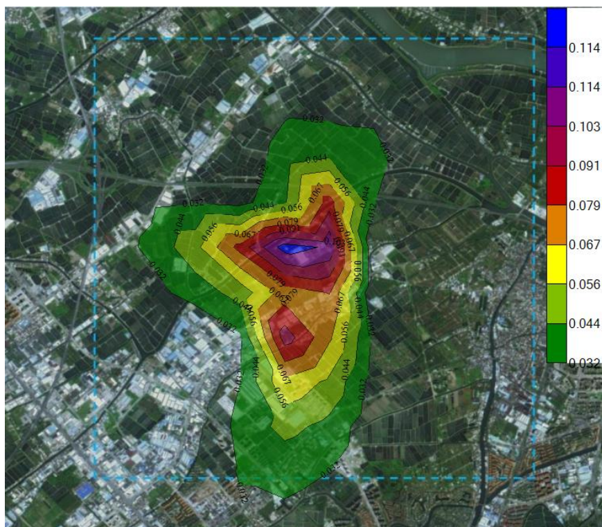
图 5-34 NO 2 叠加后 98%保证率日平均质量浓度分布图
