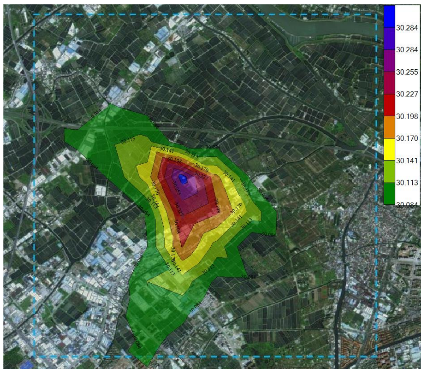
图 5-45 氯化氢叠加后 1 小时平均质量浓度最大值分布图
