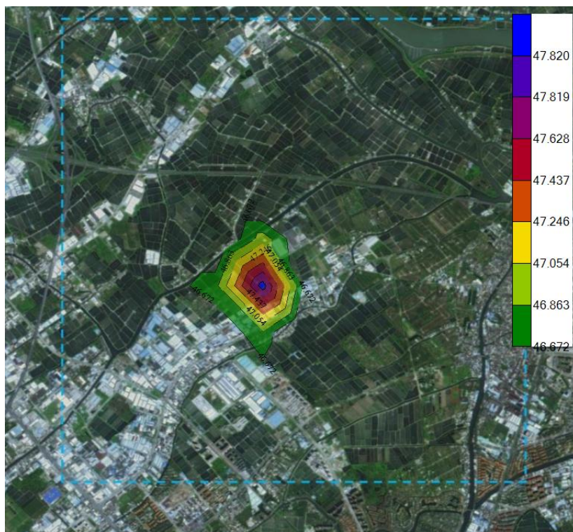
图 5-38 PM 2.5 叠加后保证率日平均质量浓度分布图
