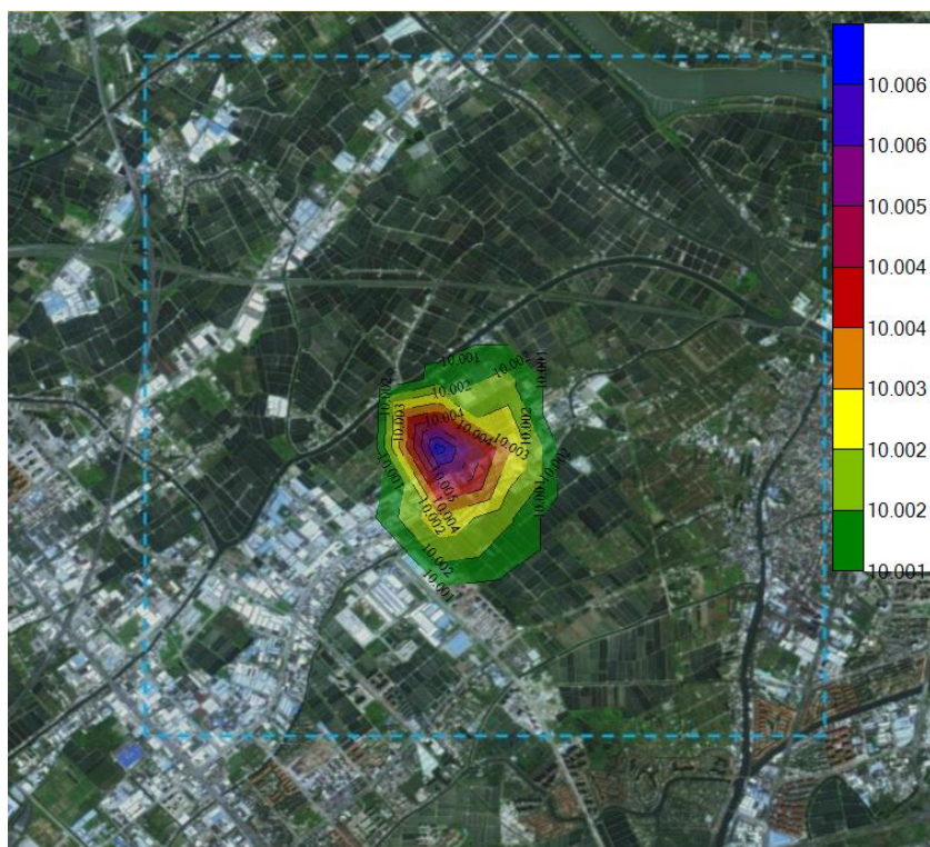
图 5-32 SO 2 叠加后保证率日平均质量浓度分布图
