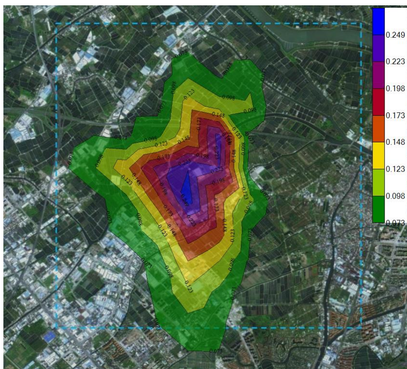
图 5-19 NO 2 新增污染源最大日平均质量浓度分布图
