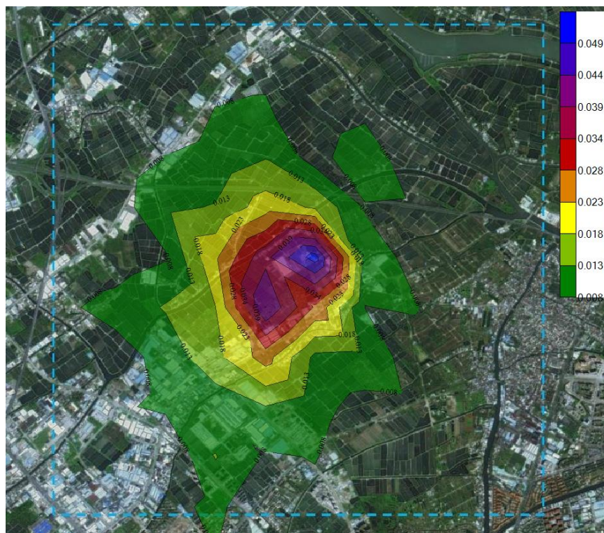
图 5-27 硫化氢新增污染源最大 1 小时质量浓度分布
