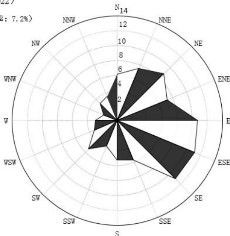
中山近二十年累年9月风向频率统计
