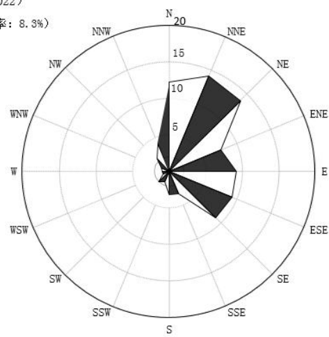
中山近二十年累年10月风向频率统计
