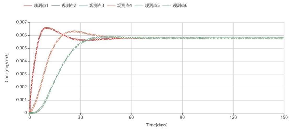
图 5-50 石油烃 (C 10 -C 40 ) 垂直入渗结果 (时间变化)
