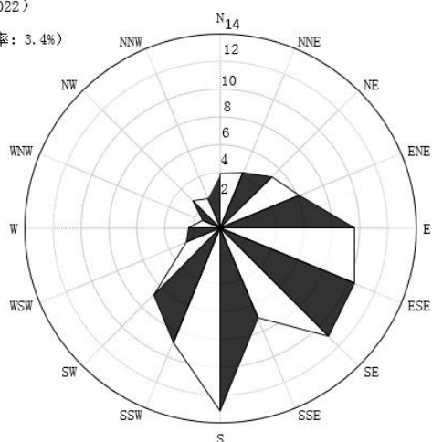
中山近二十年累年5月风向频率统计
