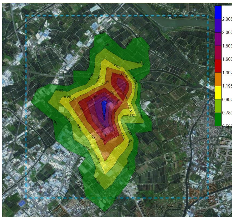
图 5-23 PM 2.5 新增污染源最大日均质量浓度分布图
