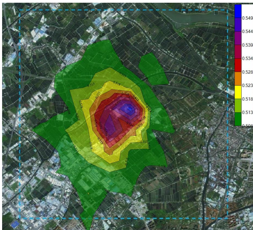
图 5-43 硫化氢叠加后 1 小时平均质量浓度最大值分布图
