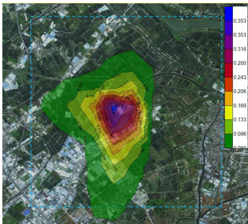
图 5-22 PM_{10} 新增污染源最大年平均质量浓度分布图
