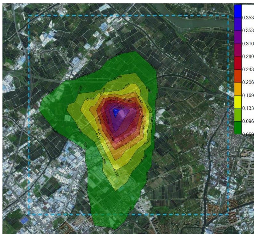
图 5-37 PM_{10} 叠加后年平均质量浓度分布图
