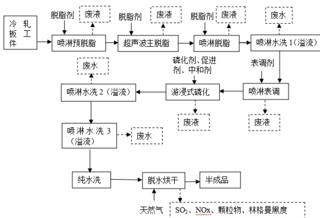
图 3-12 磷化处理线生产工艺流程及产污节点图
