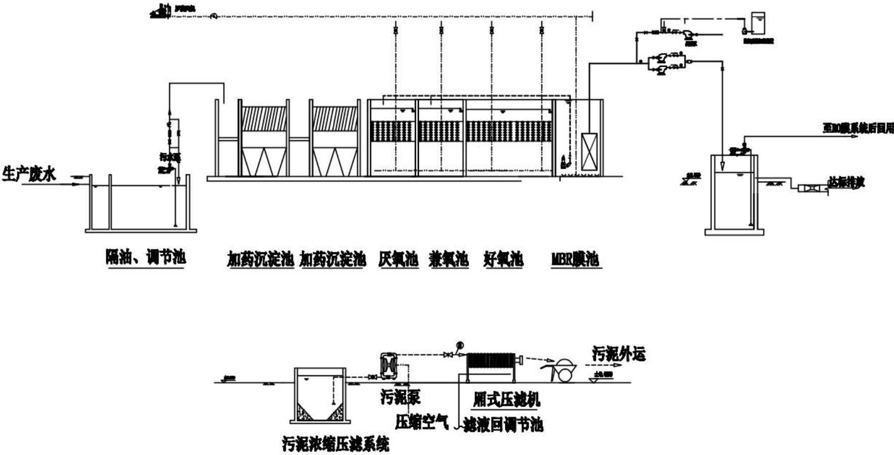
图 6-3 厂房 2F 污水处理站设计图
