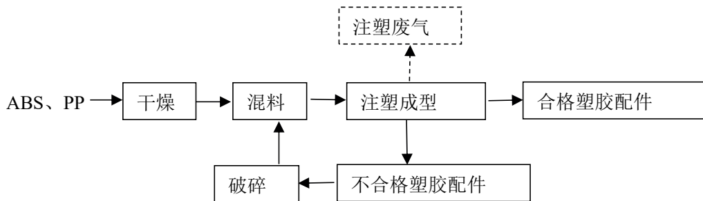
图 3-15 塑胶配件生产工艺及产污节点图
