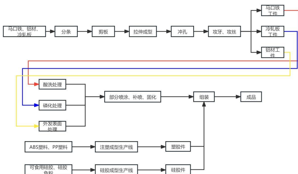
图 3-10 项目总生产工艺流程图
