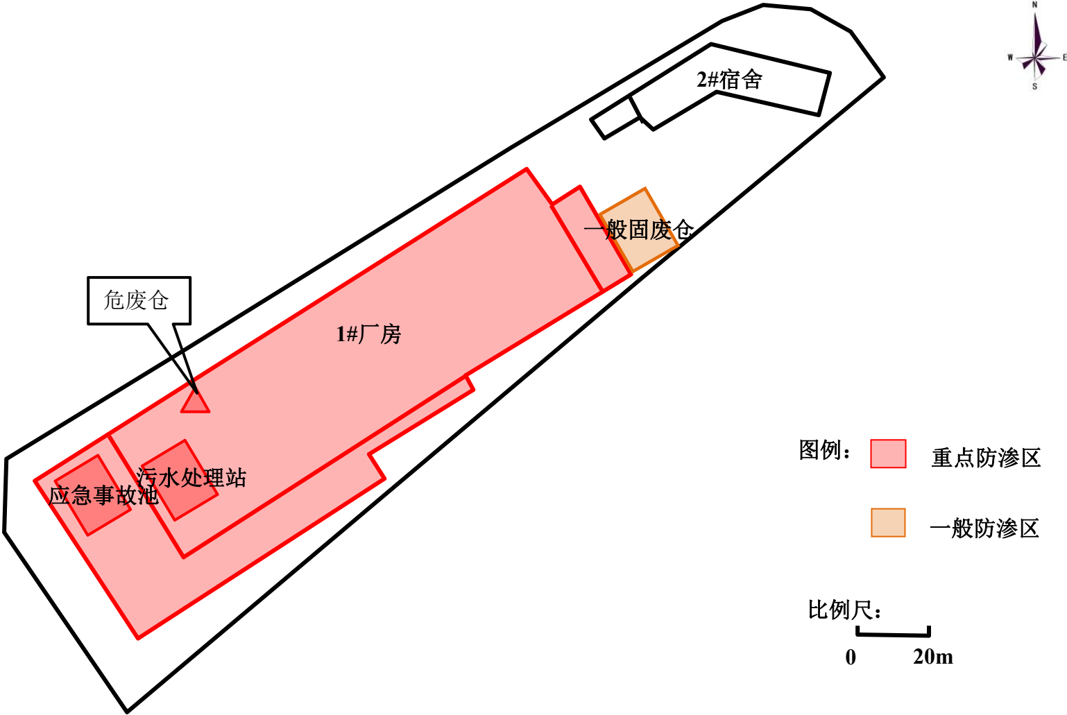
图 5-49 项目地下水分区防渗图
