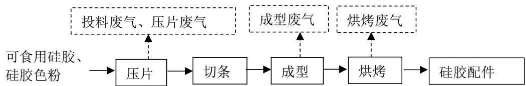
图 3-16 硅胶配件生产工艺及产污节点图
