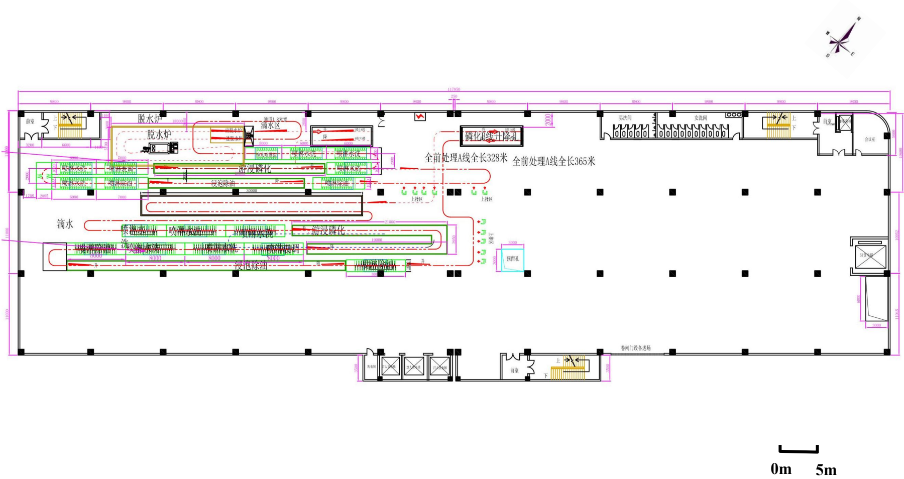
图 3-6 项目生产车间第 5 层平面布置图
