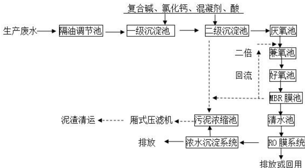
图 6-1 生产废水处理流程图
