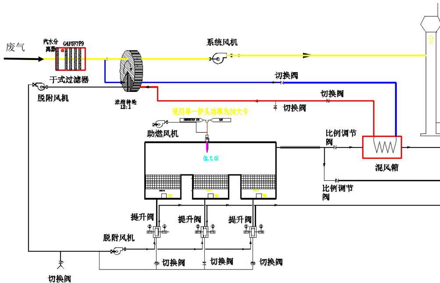
图 6-5 工艺流程示意图
