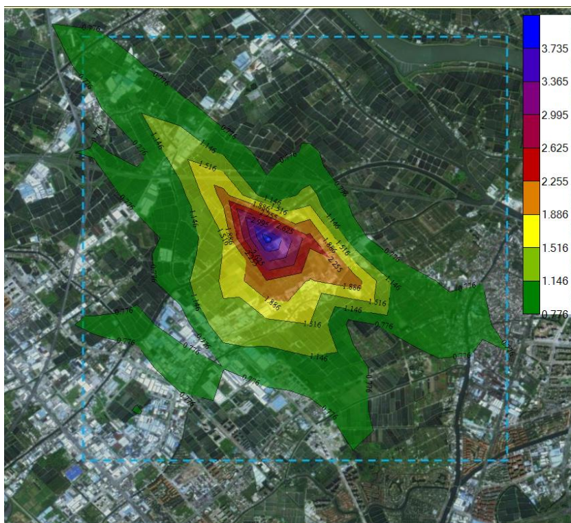
图 5-18 NO 2 新增污染源最大小时质量浓度分布图
