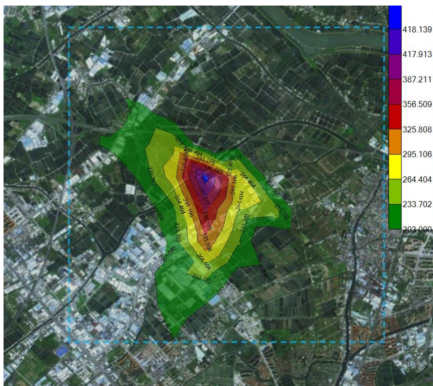
图 5-41 NMHC 叠加后 1 小时平均质量浓度最大值分布图
