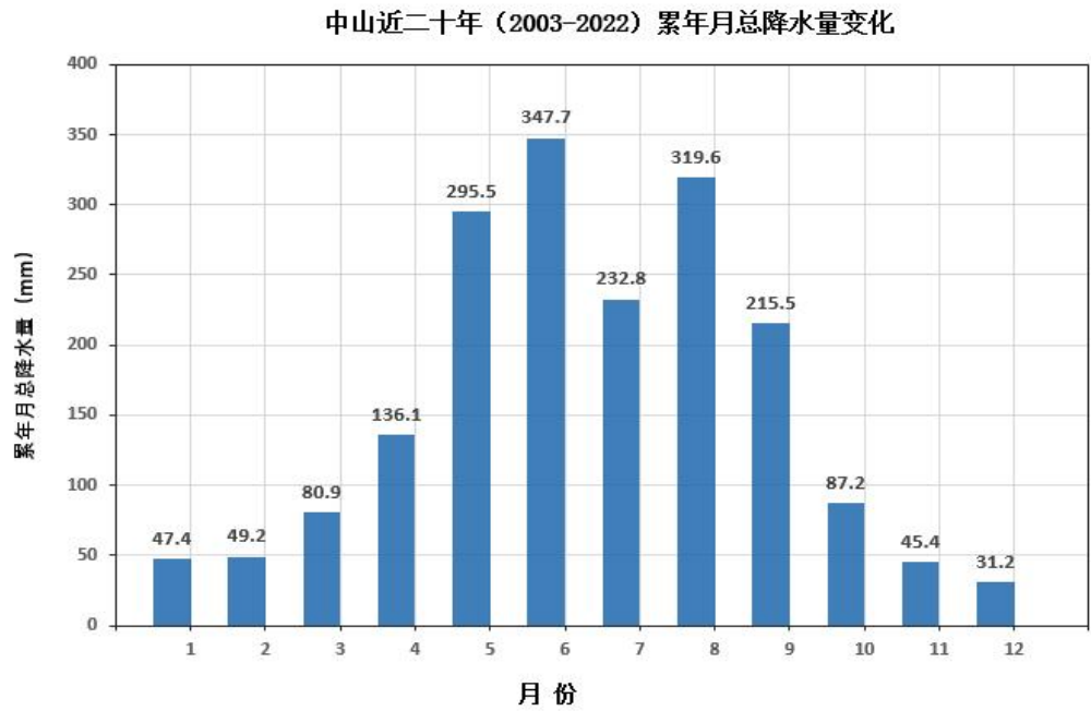
图 5-4 中山气象站月总降水量变化（统计年限：2003-2022 年）
