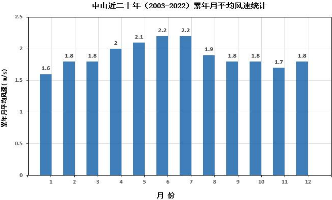
图 4-2 中山市 2003~2022 年逐月平均风速变化曲线
