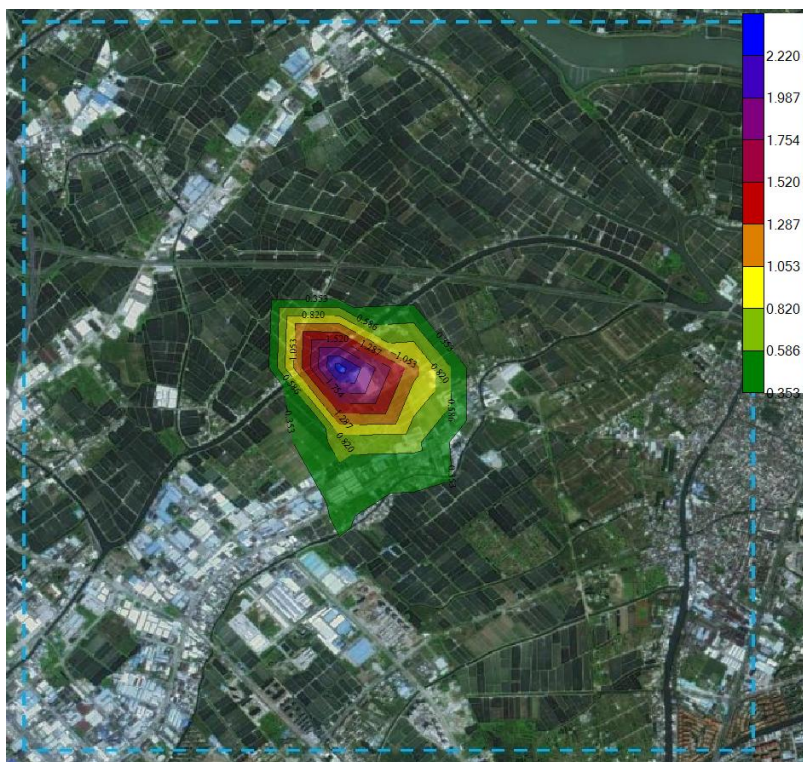
图 5-40 TSP 叠加后日平均质量浓度分布图
