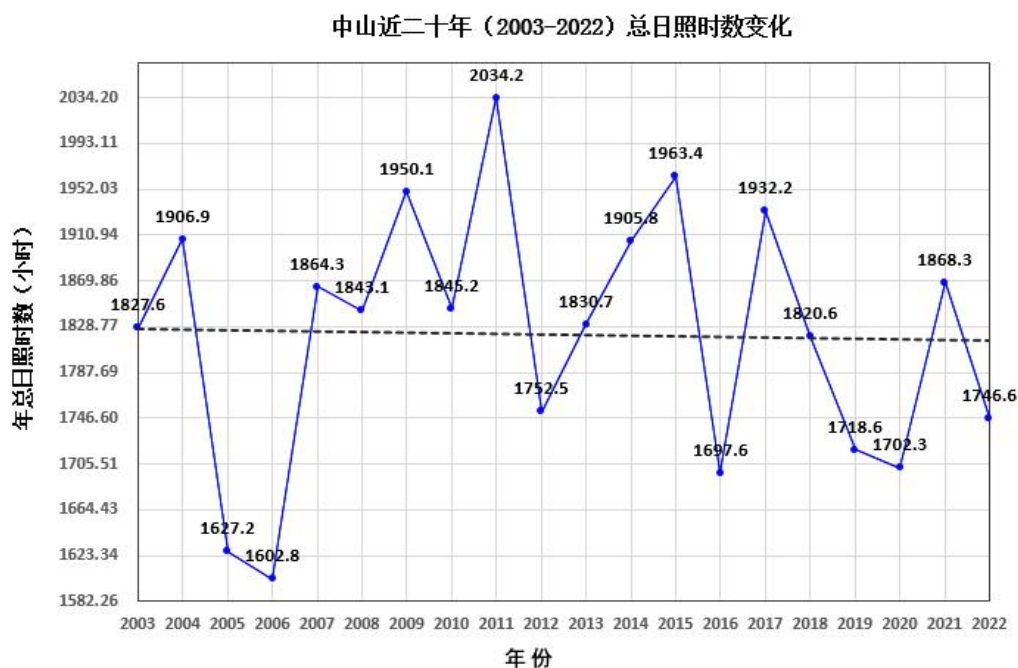
图 4-8 中山气象站年平均日照时数变化（统计年限：2003-2022 年）
