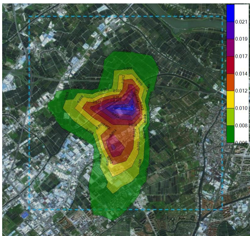
图 5-15 SO 2 新增污染源最大小时质量浓度分布图
