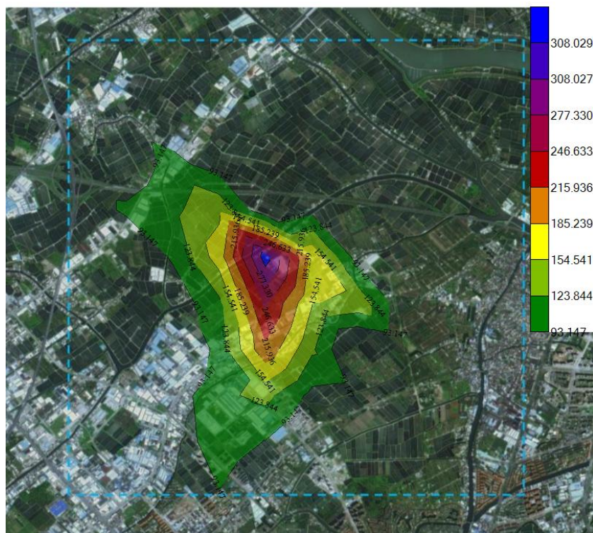
图 5-30 NMHC 新增污染源最大小时质量浓度分布图
