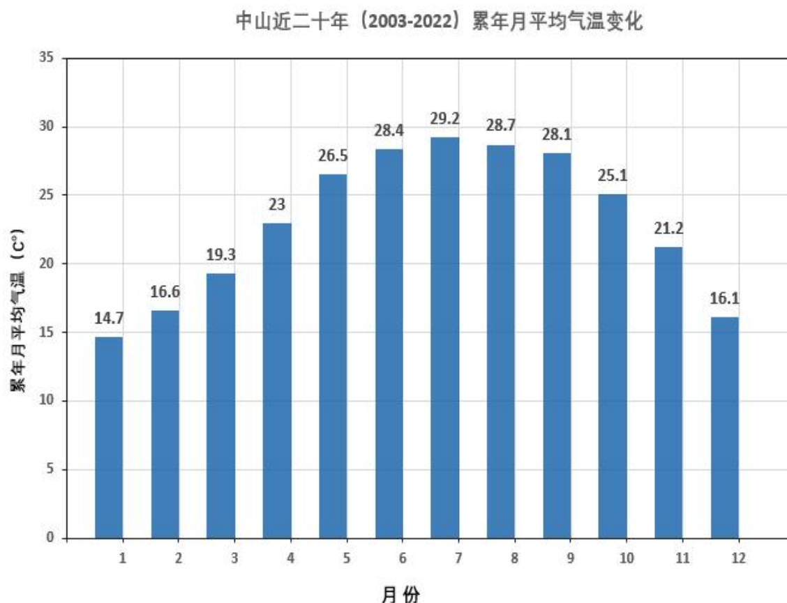
图 5-1 中山市 2003~2022 年逐月平均气温变化曲线
