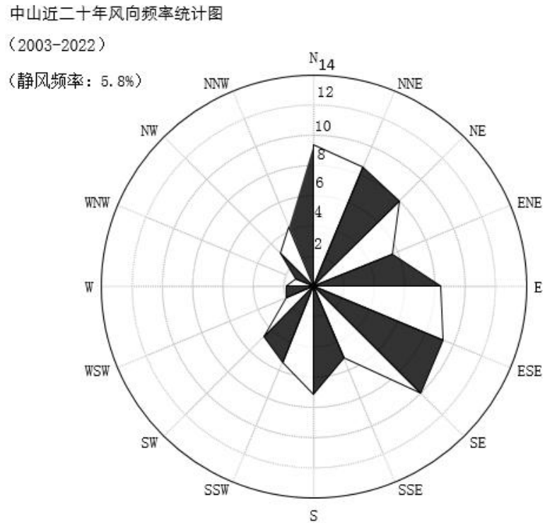
图 5-3 中山气象站风向玫瑰图（统计年限：2003-2022 年）
