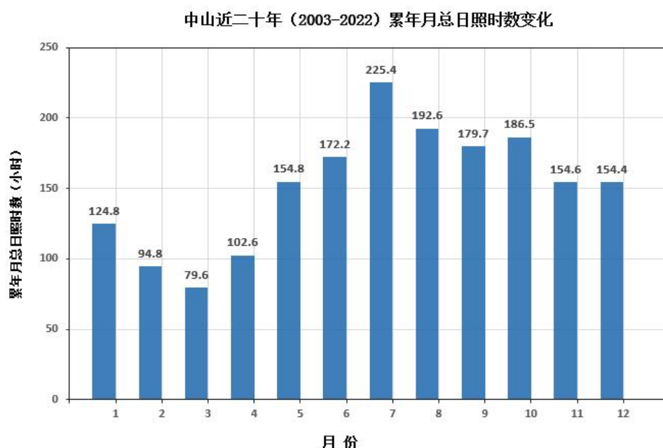
图 5-6 中山气象站月平均日照时数变化（统计年限：2003-2022 年）
