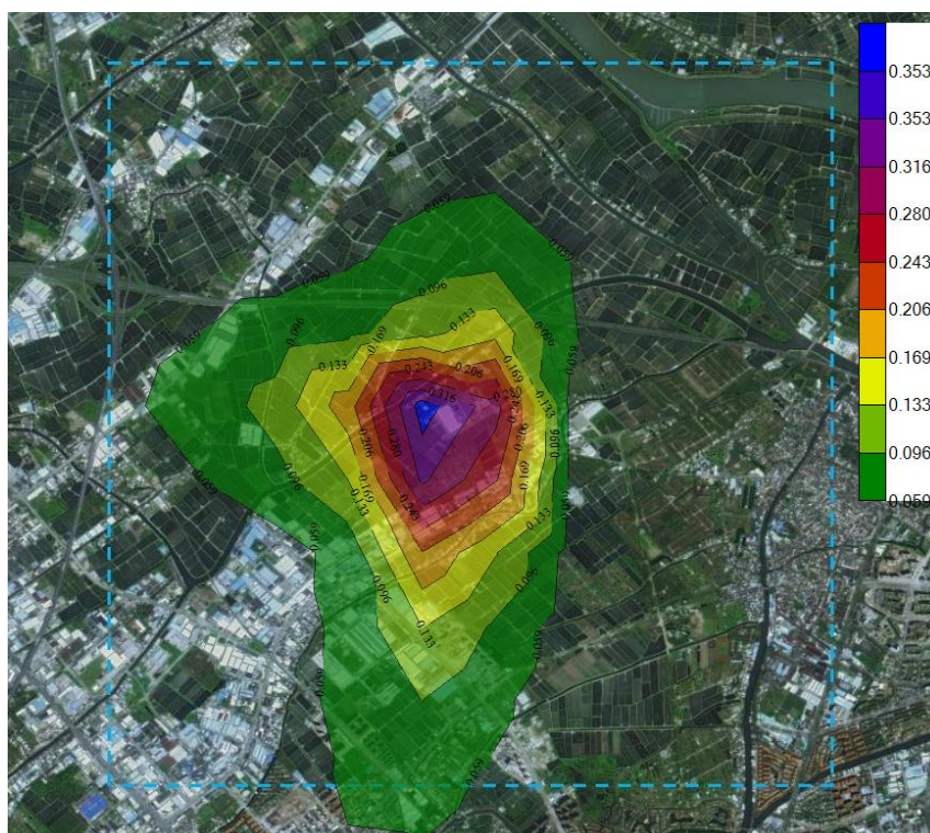
图 5-24 PM 2.5 新增污染源最大年平均质量浓度分布图
