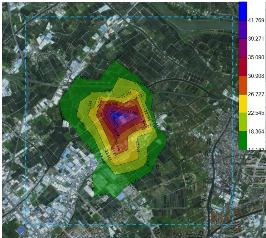
图 5-31 TVOC 新增污染源最大 8 小时质量浓度分布图
