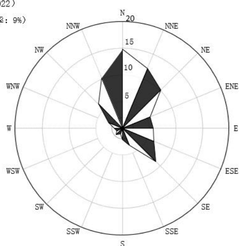
中山近二十年累年1月风向频率统计
