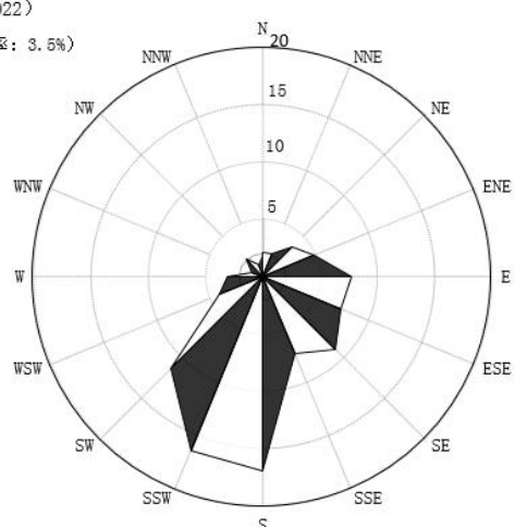
中山近二十年累年6月风向频率统计
