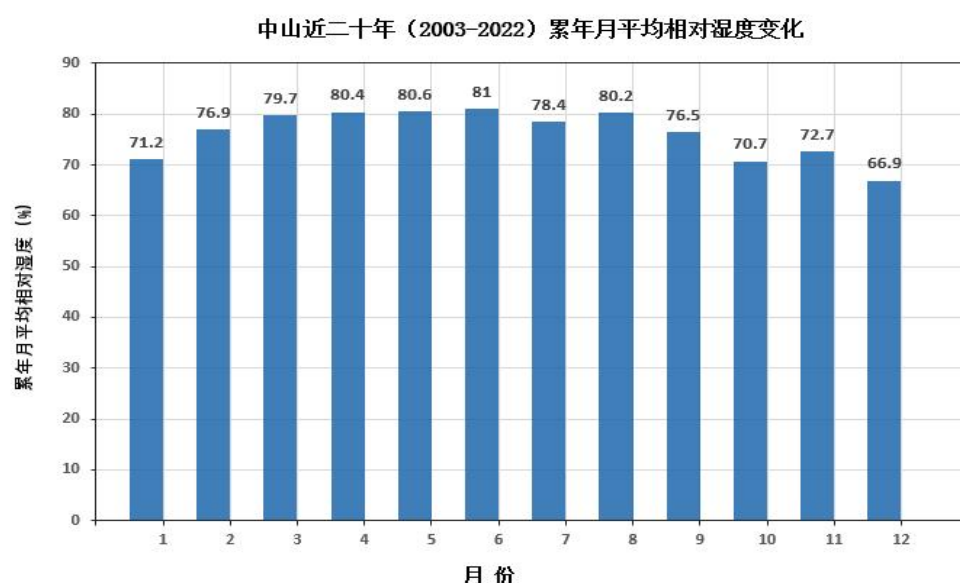
图 5-5 中山气象站月平均相对湿度变化（统计年限：2003-2022 年）
