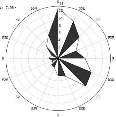
中山近二十年累年4月风向频率统计
