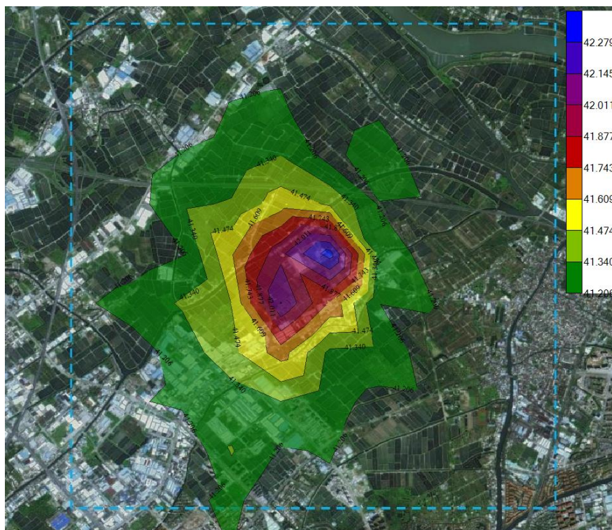
图 5-44 氨气叠加后 1 小时平均质量浓度最大值分布图
