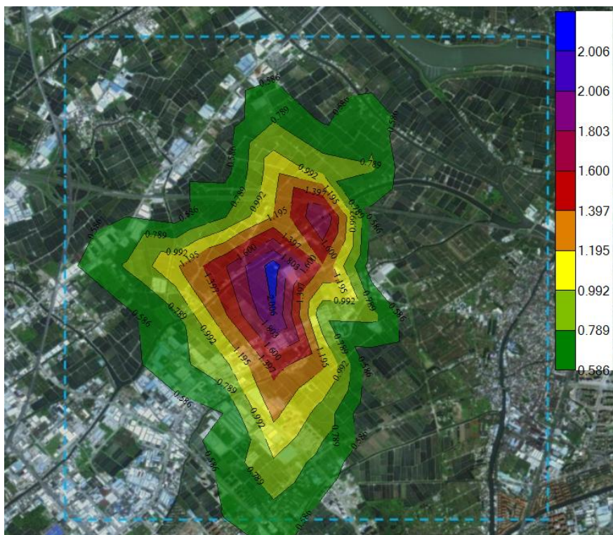
图 5-21 PM_{10} 新增污染源最大日平均质量浓度分布图
