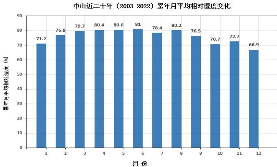
图 4-5 中山气象站月平均相对湿度变化（统计年限：2003-2022 年）
