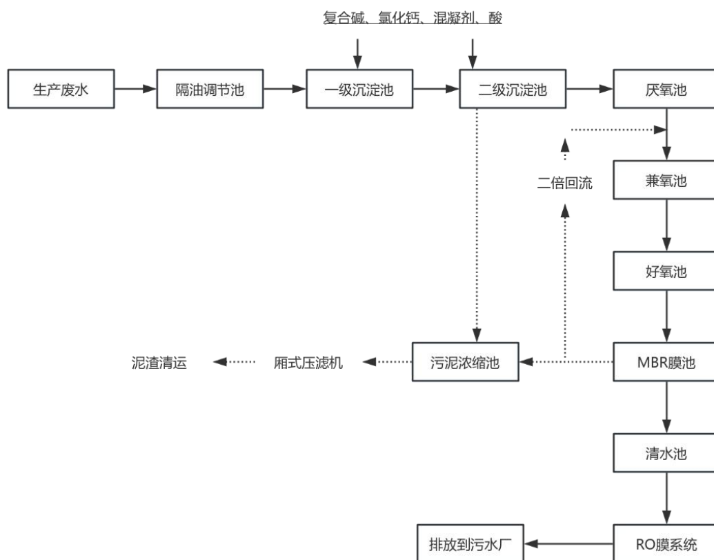
图 3-18 生产废水处理流程图
