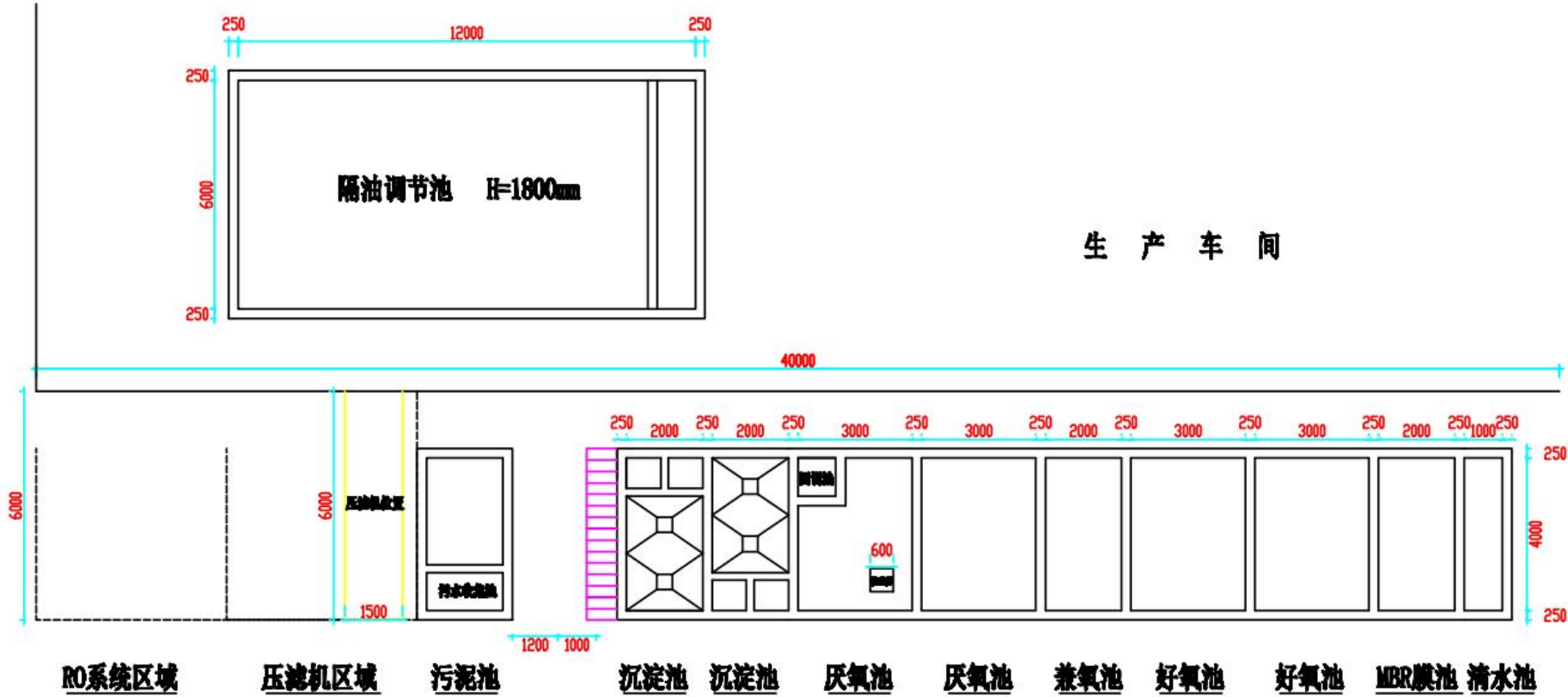
图 6-2 厂房 1F 污水处理站分布图
