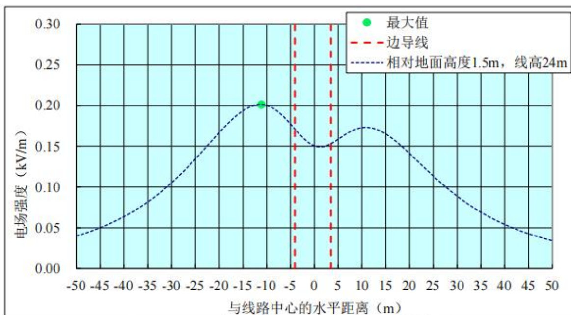
图8.2-6 工频电场强度预测结果衰减趋势线图
