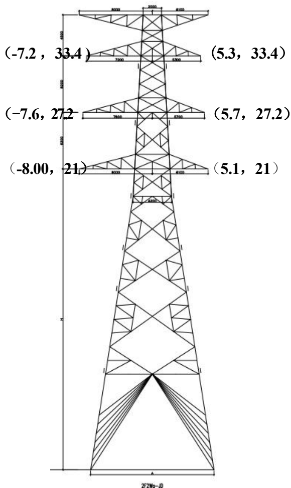
220kV杆塔
