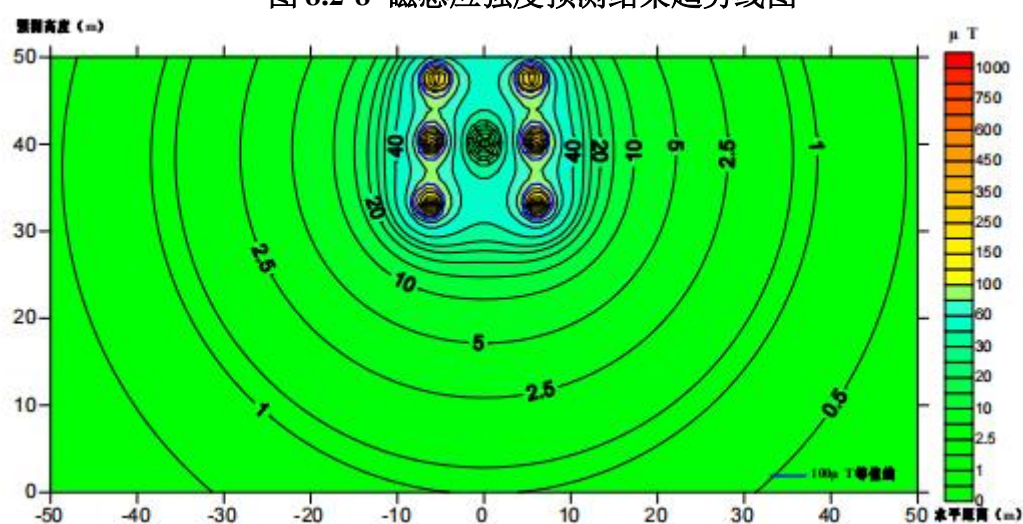
图 8.2-8 磁感应强度预测结果趋势线图
