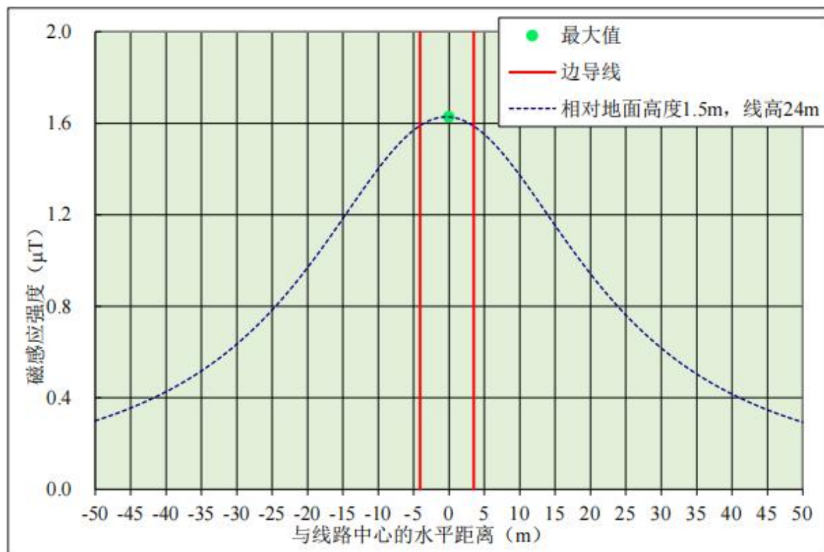
图 8.2-10 磁感应强度预测结果趋势线图
