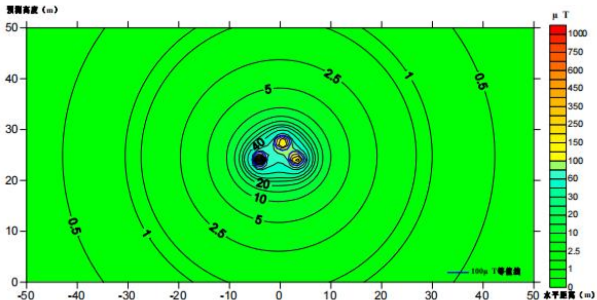
图 8.2-11 磁感应强度预测结果等值线图
