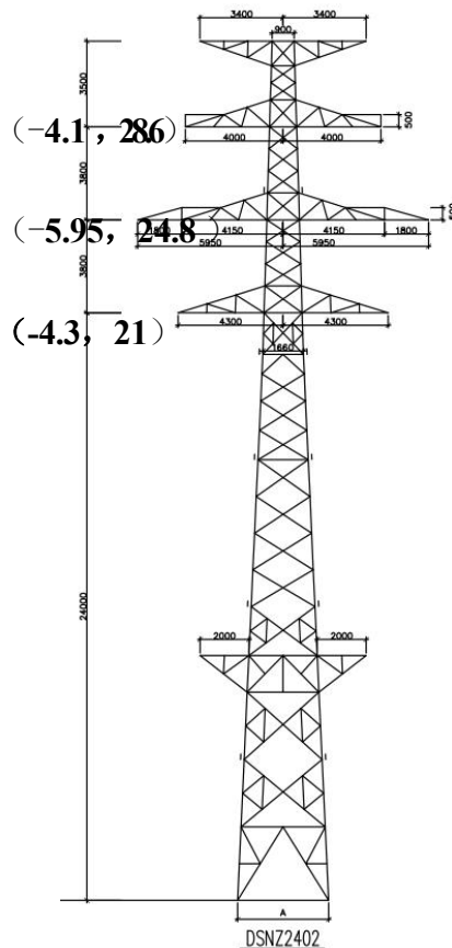
110kV杆塔
