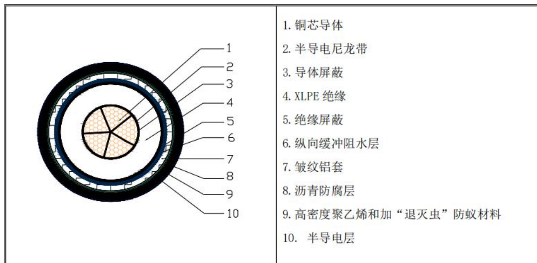
图2-1 电缆截面图
