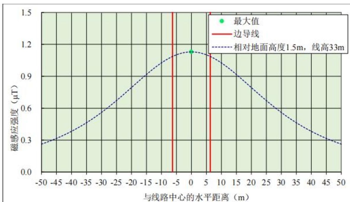
图 8.2-8 磁感应强度预测结果趋势线图
