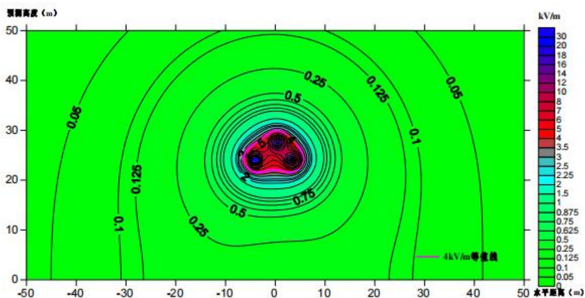
图 8.2-7 工频电场强度预测结果等值线图
