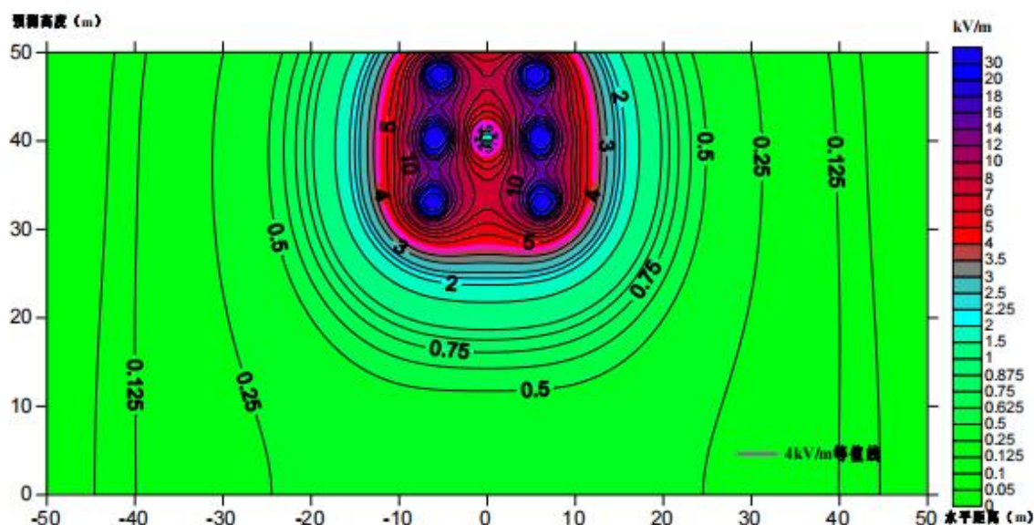
图 8.2-5 工频电场强度预测结果等值线图
