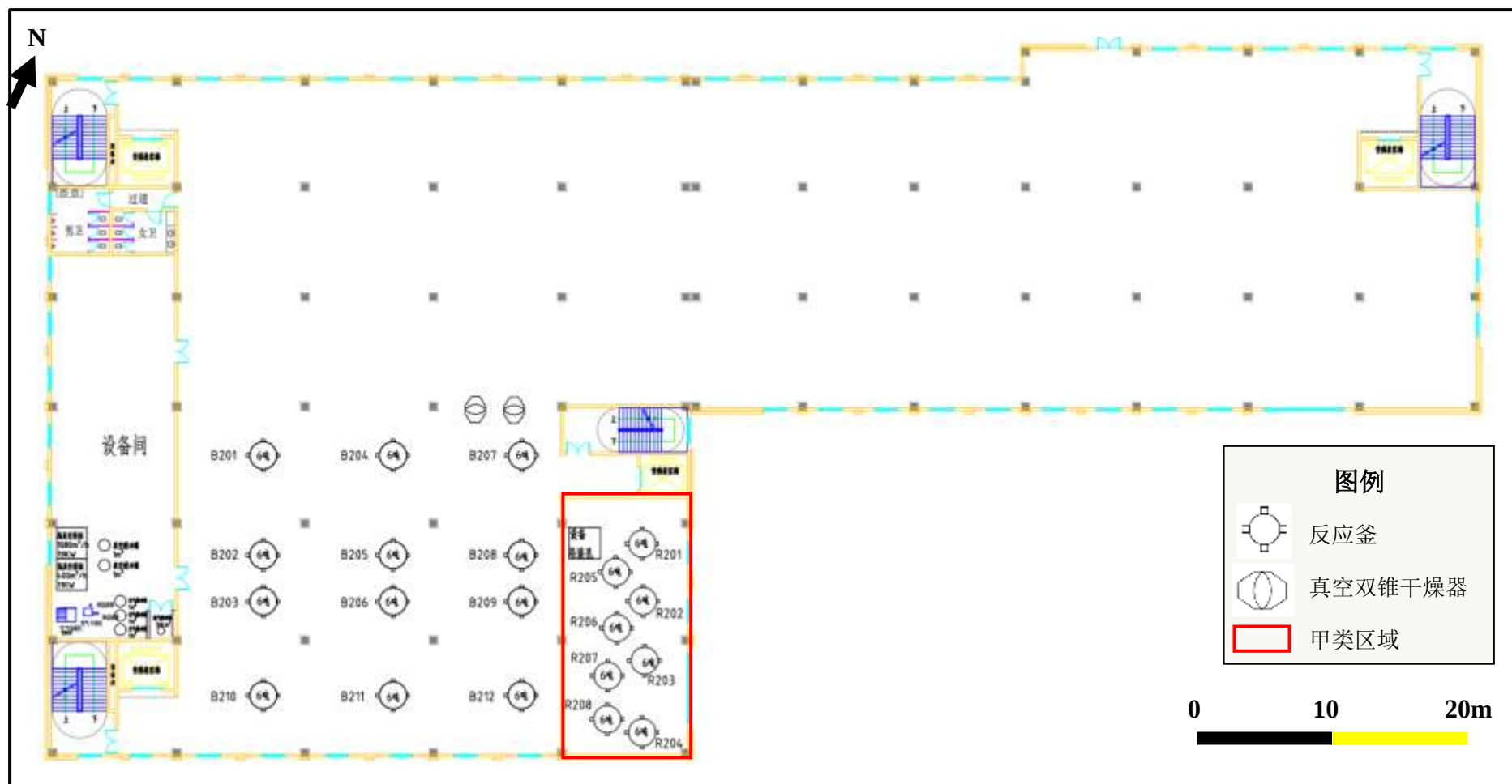
图3.5-3 厂房B车间平面布置图（2层）
