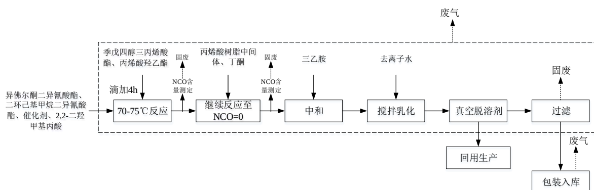
图 4.3-16 水性聚氨酯丙烯酸酯树脂乳液工艺流程及产污环节
