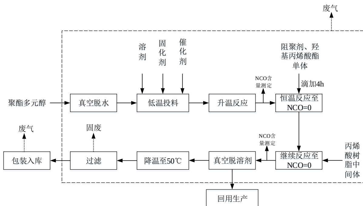
图4.3-3 聚氨酯丙烯酸酯树脂中间体工艺流程及产污环节
