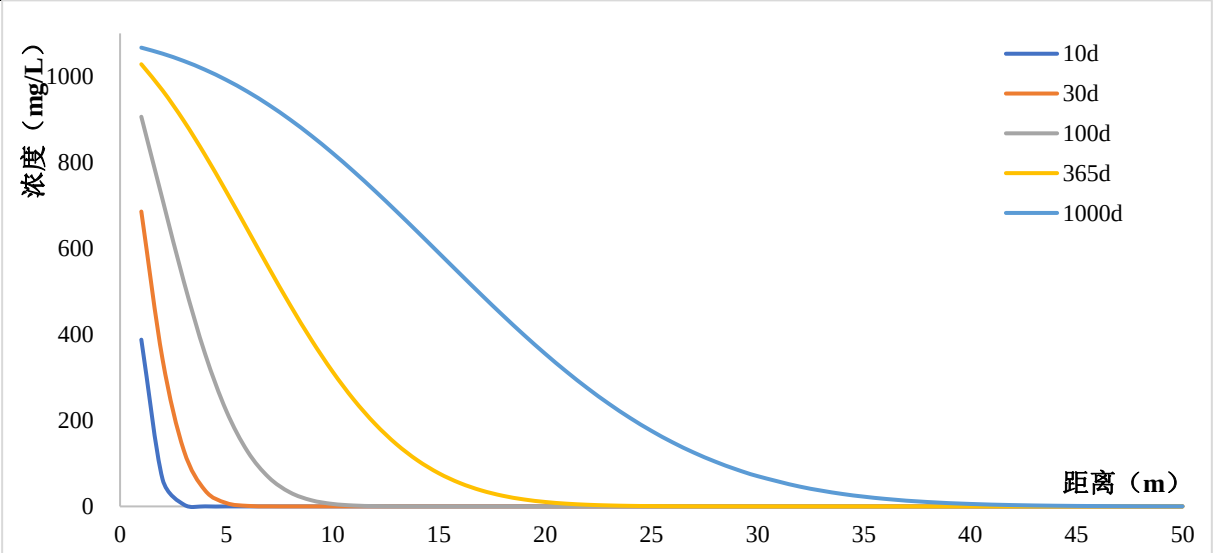
图7.3-6 不同时段COD Mn 运移影响范围图
