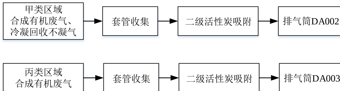
图8.3-1 废气处理流程图
