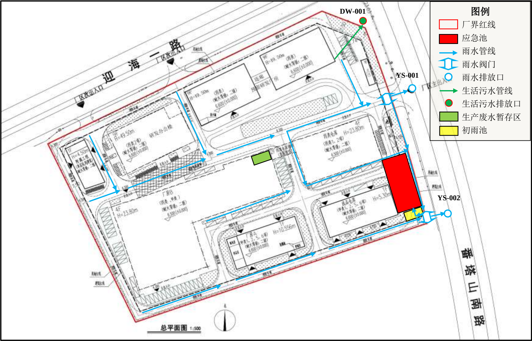
图3.5-4 厂区雨污管网图
