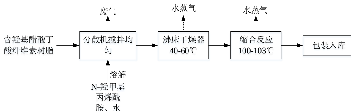
图 4.3-13 可 UV 固化纤维素树脂工艺流程及产污环节
