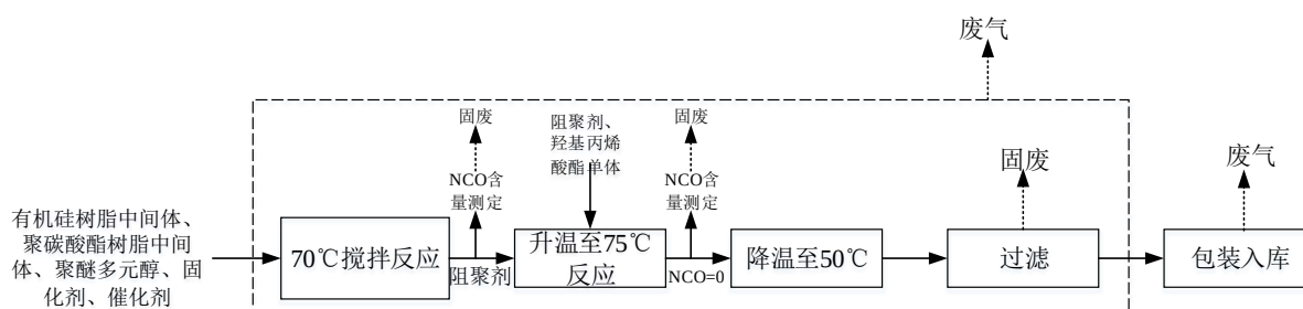
图 4.3-31 有机硅改性聚氨酯丙烯酸酯树脂工艺流程及产污环节
