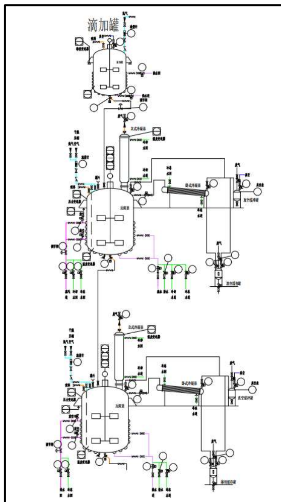
图4.3-15 水性聚氨酯树脂乳液生产设备连接示意图
