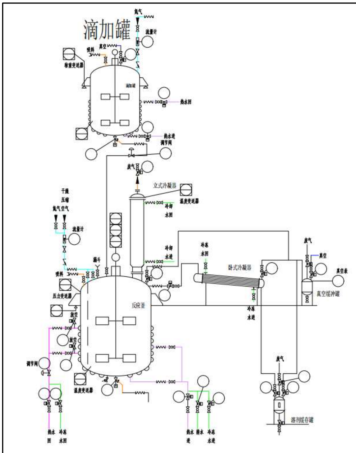
图4.3-26 水性聚氨酯丙烯酸酯树脂乳液生产设备连接示意图
