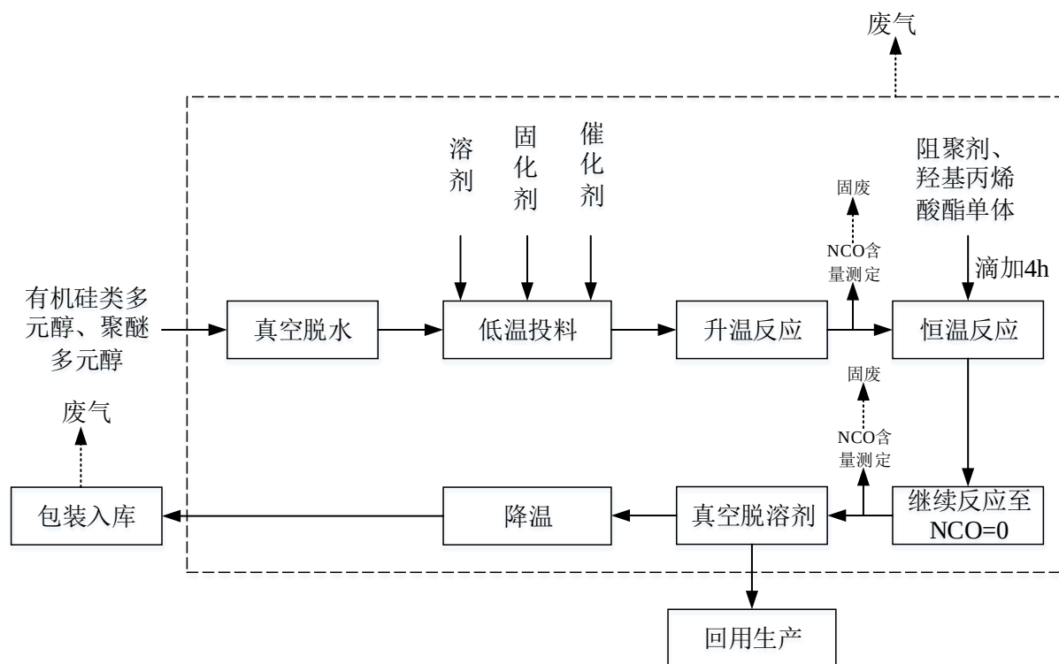
图4.3-5 有机硅树脂中间体工艺流程及产污环节
