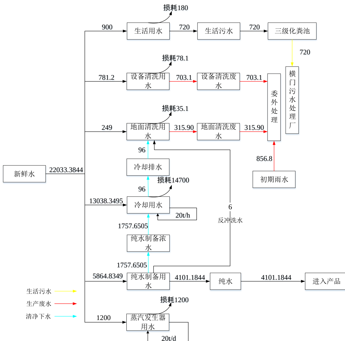
图3.8-1 本项目水平衡图 单位: t/a
