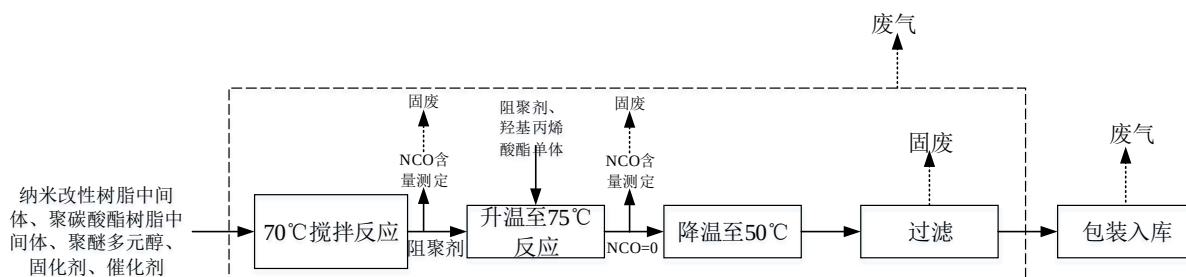
图 4.3-29 纳米改性聚氨酯丙烯酸酯树脂工艺流程及产污环节
