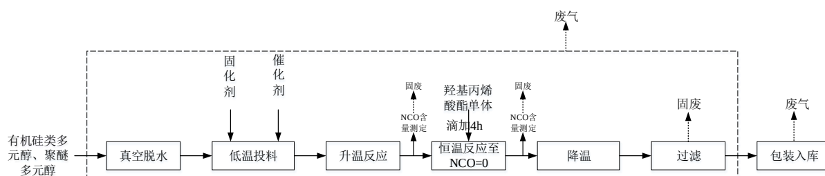
图 4.3-21 有机硅改性聚氨酯丙烯酸酯树脂（无溶剂法）工艺流程及产污环节
