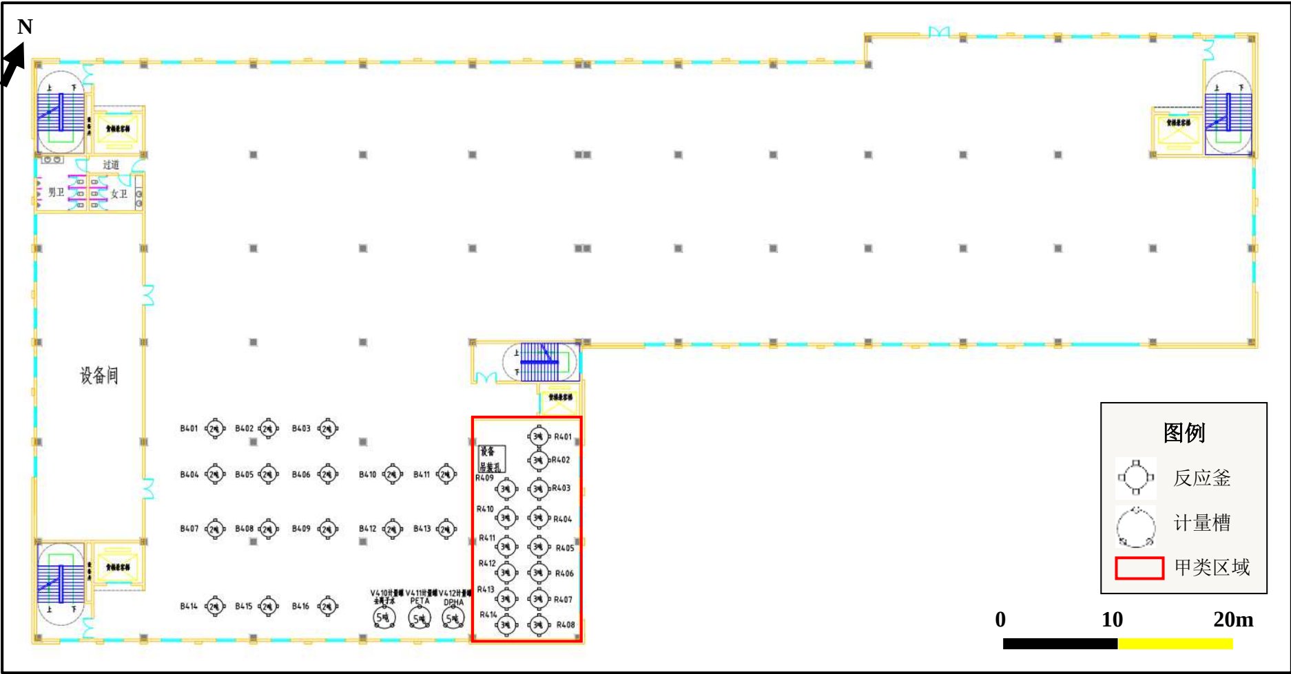
图3.5-3 厂房B车间平面布置图（4层）
