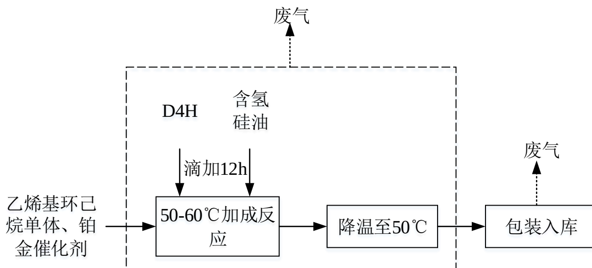
图 4.3-9 UV 固化阳离子有机硅树脂工艺流程及产污环节
