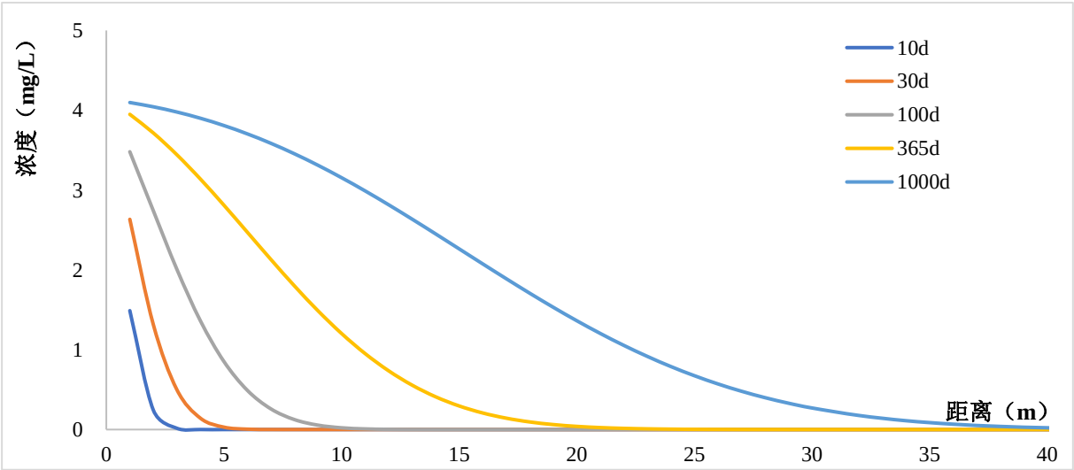
图7.3-7 不同时段氨氮运移影响范围图
