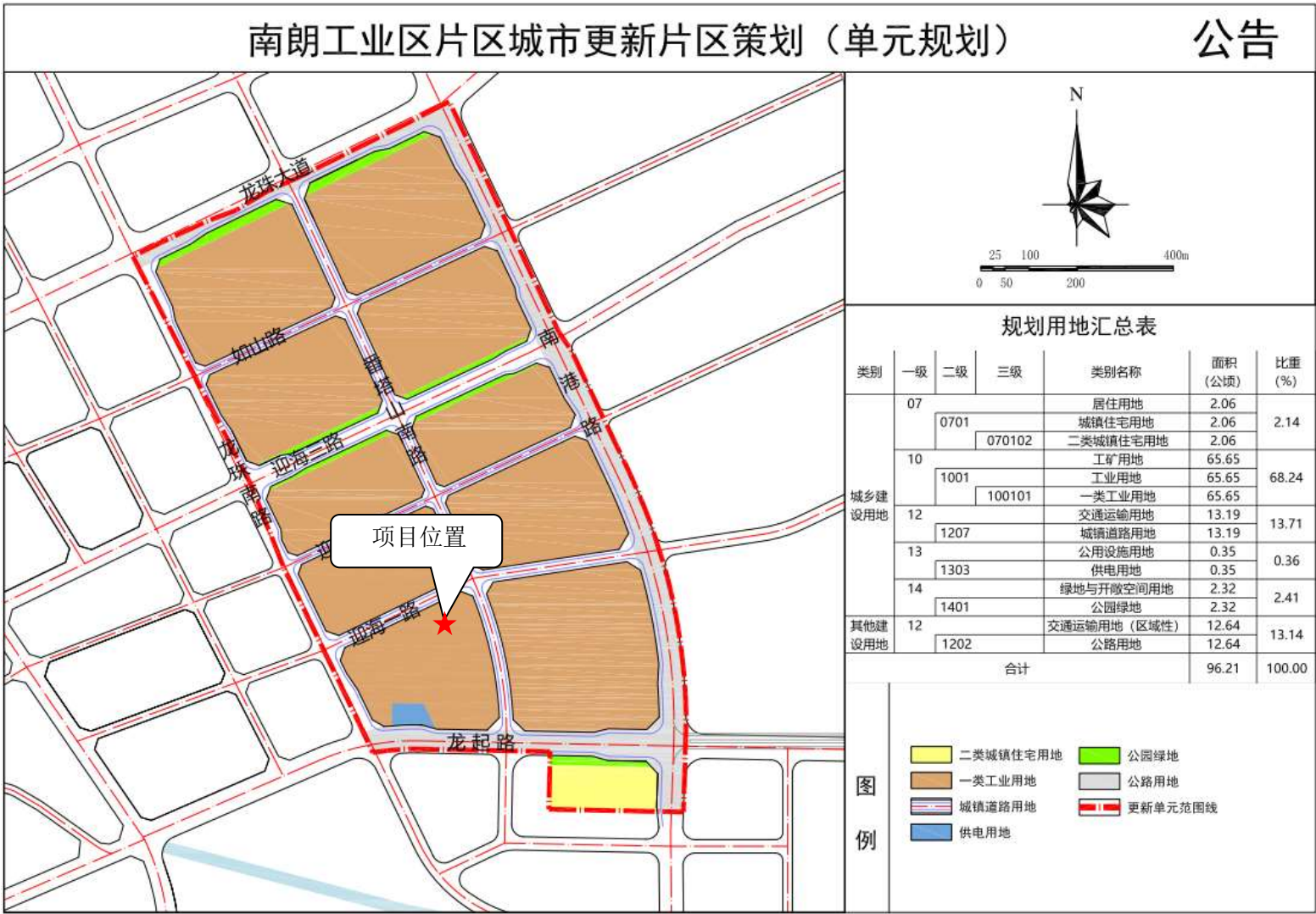
图 1.3-1 中山市南朗工业片区城市更新片区策划（单元规划）
