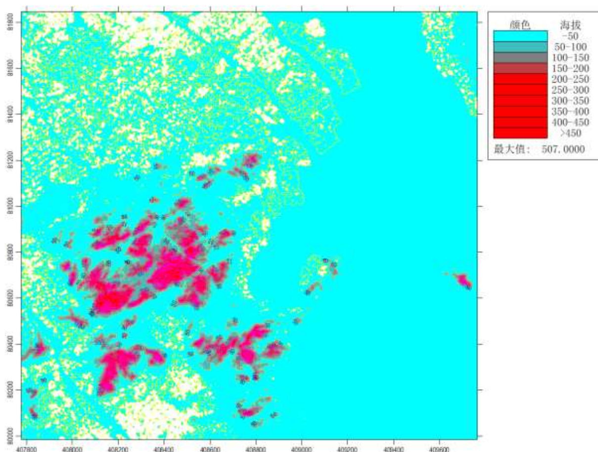
图 7.4-15 项目周边地形高程分布图
