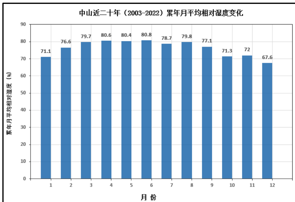
图7.4-10 中山基本站月平均相对湿度（纵轴为百分比）
