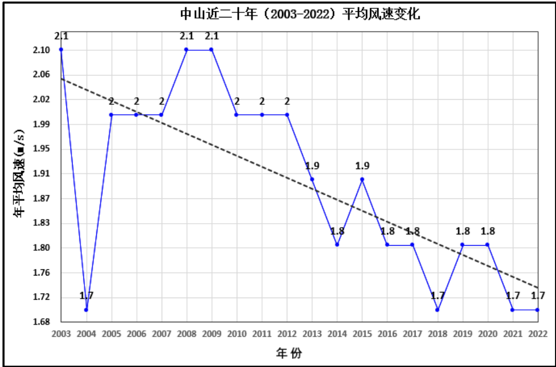
图7.4-3 中山基本站年平均风速（单位：m/s，虚线为趋势线）
