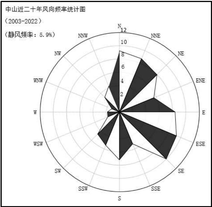
图7.4-1 中山风向玫瑰图（静风频率5.9%）
