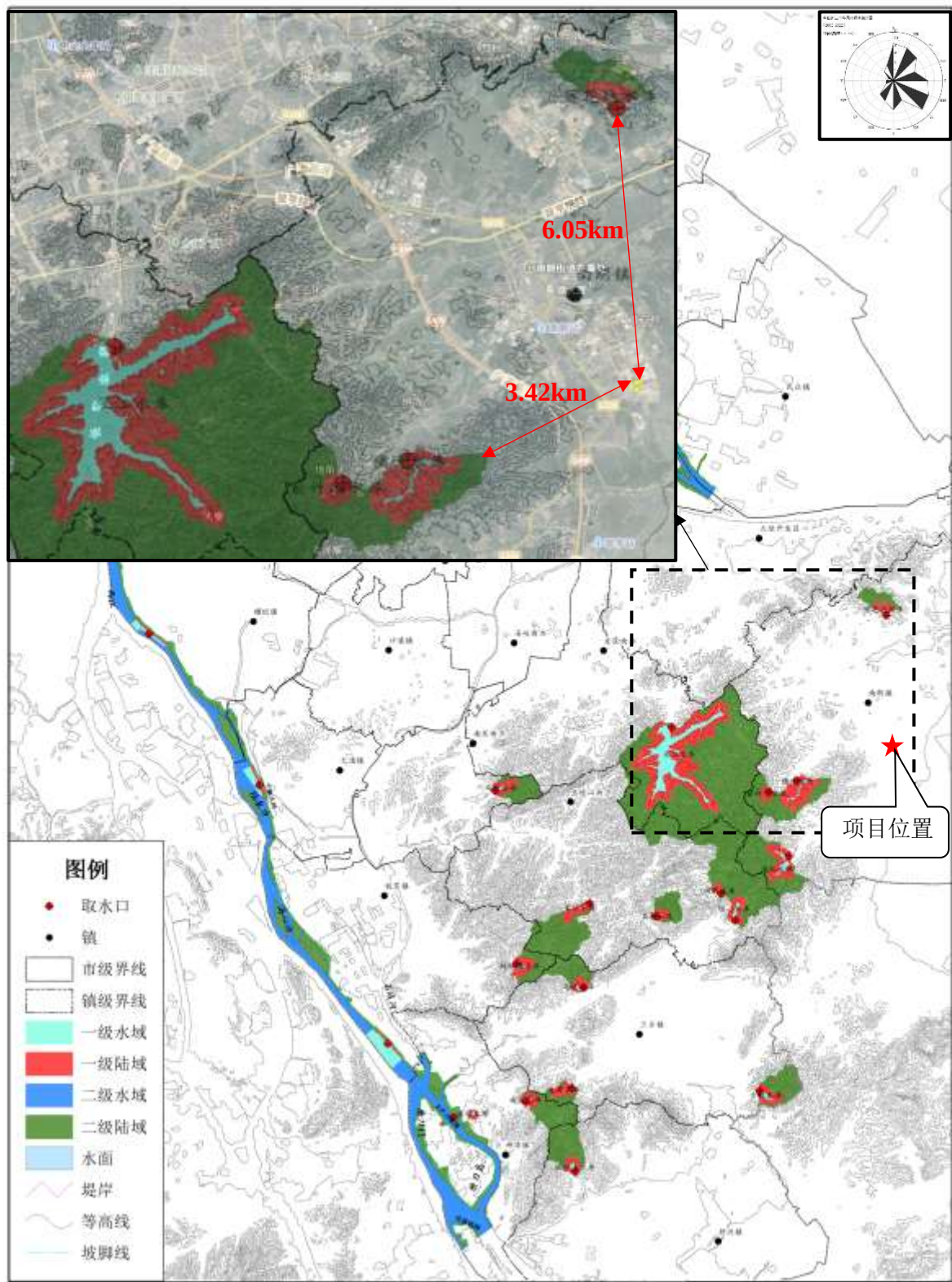
图 2.5-4 项目与饮用水源保护区的位置关系图
