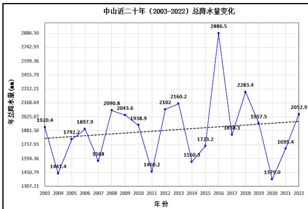
图7.4-7 中山基本站年总降水量（单位：毫米，虚线为趋势线）
