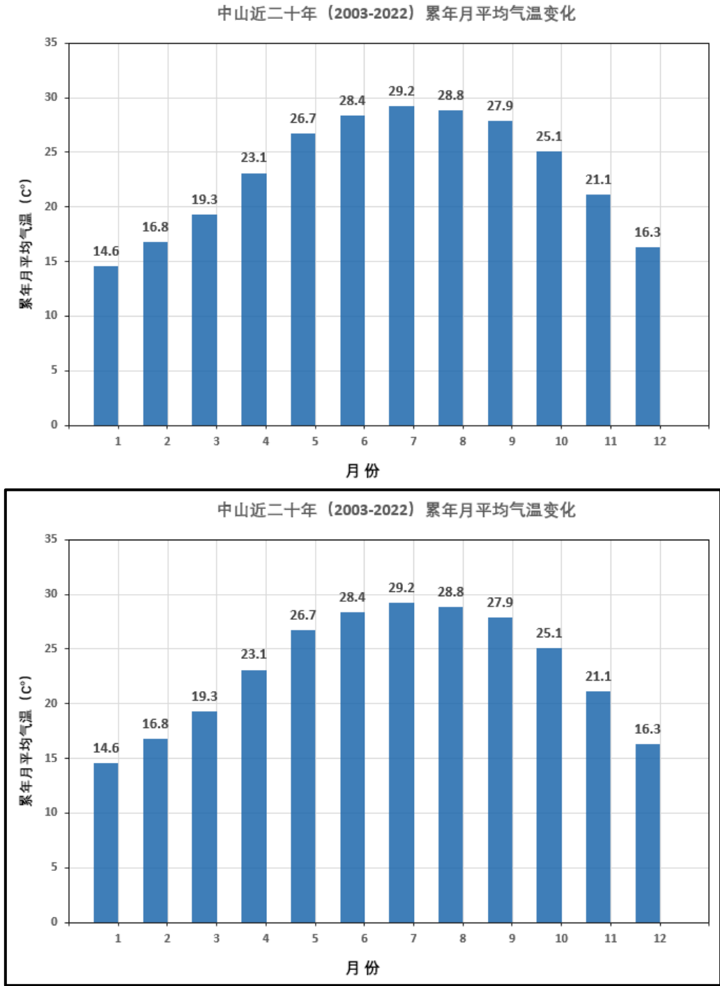
图7.4-4 中山基本站月平均气温（单位：℃）
