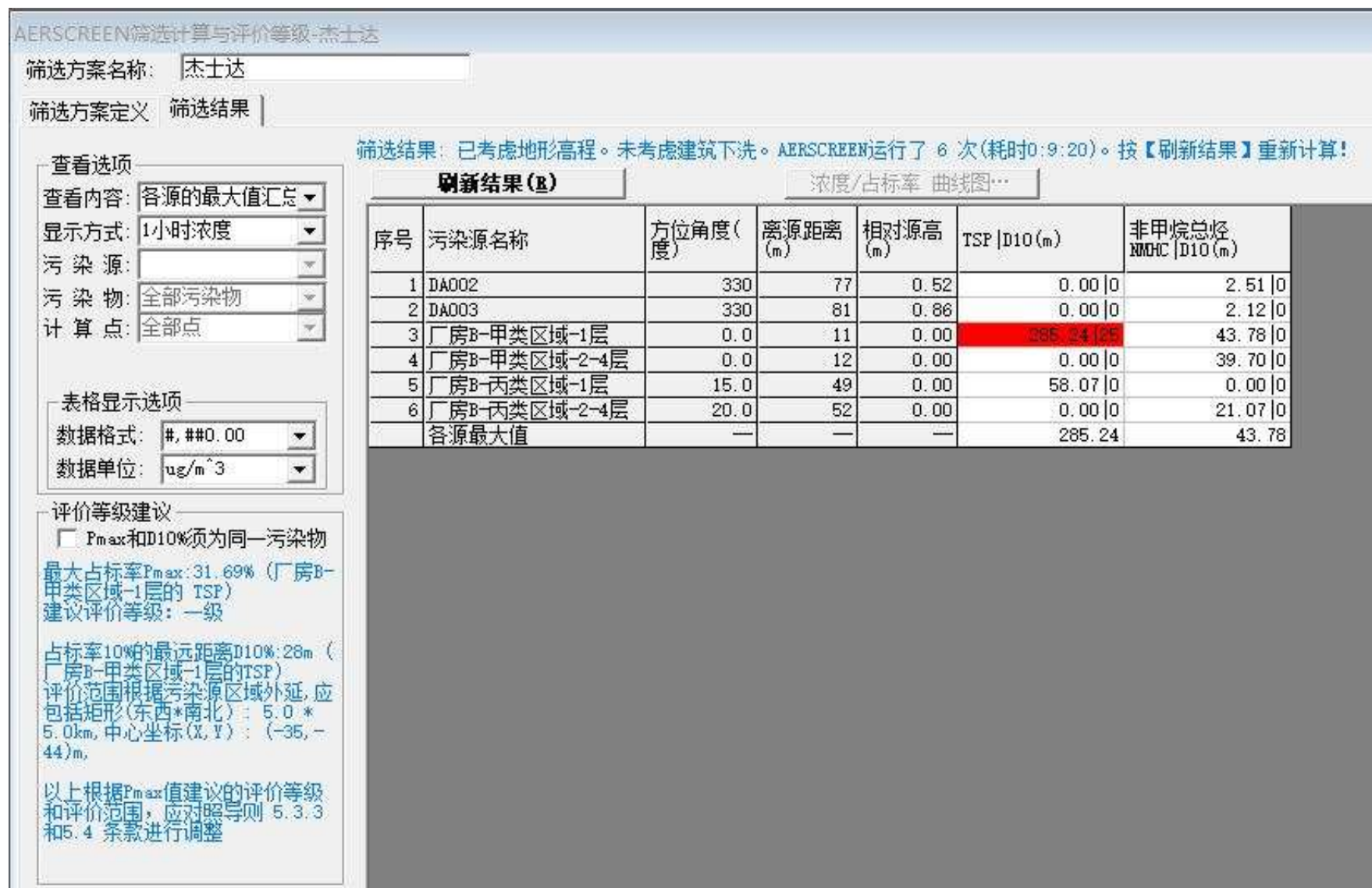
图7.4-13 本项目各污染源1h浓度最大值
