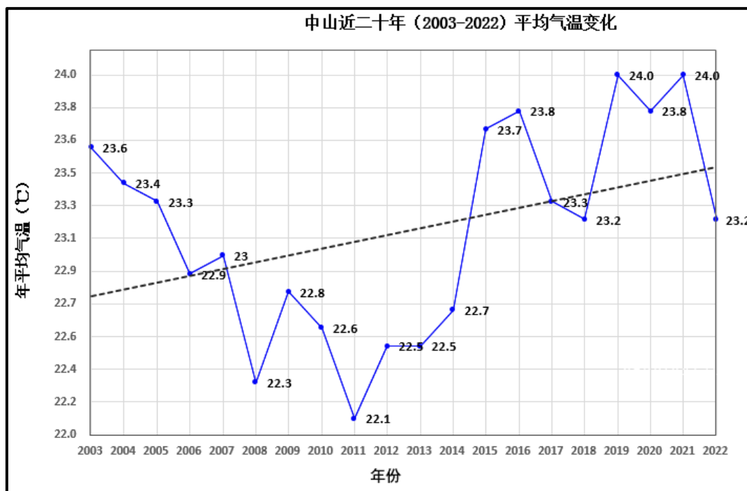
图7.4-5 中山基本站年平均气温（单位：℃，虚线为趋势线）
