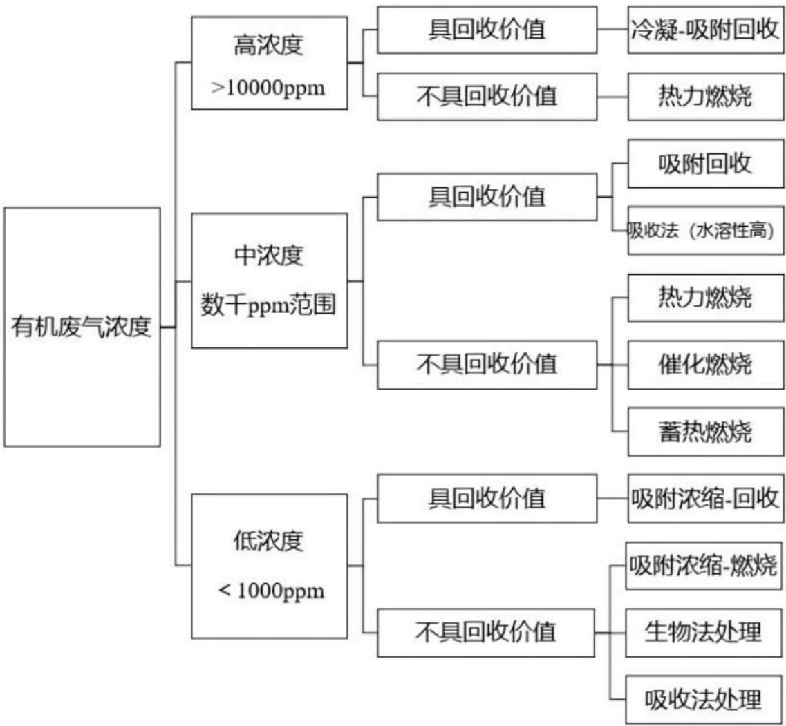
图8.3-1 VOCs治理技术适用范围（浓度）
