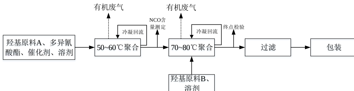
图 3.1-1 聚氨酯树脂生产工艺流程
