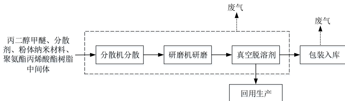
图 4.3-7 纳米改性树脂中间体工艺流程及产污环节
