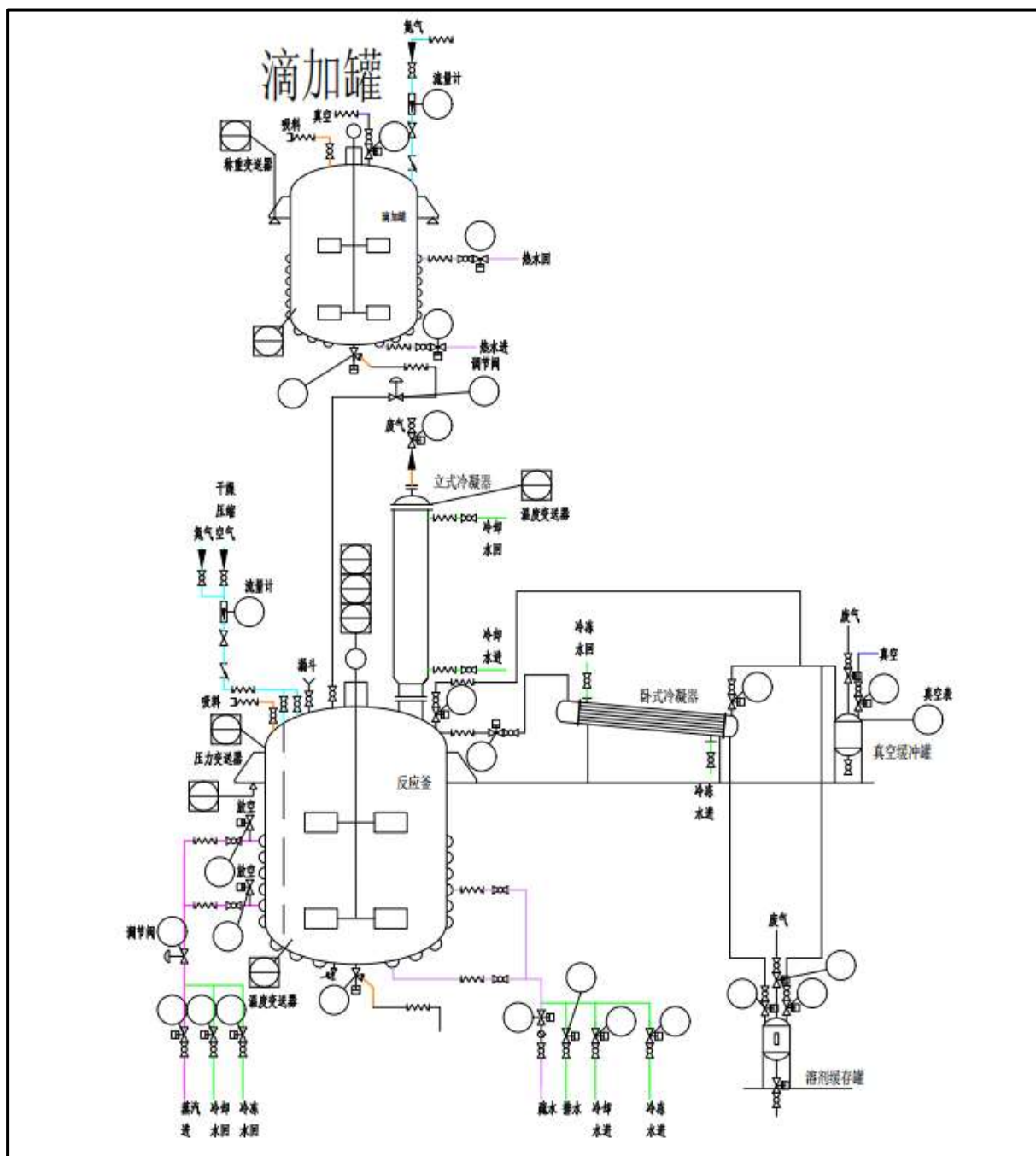
图4.3-30 纳米改性聚氨酯丙烯酸酯树脂生产设备连接示意图
