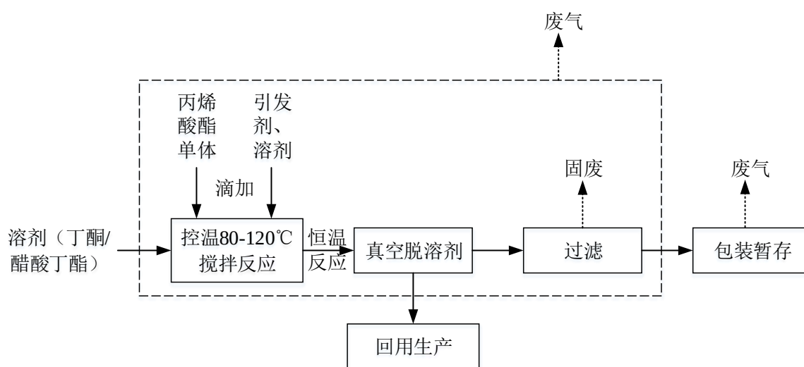
图4.3-1 丙烯酸树脂中间体工艺流程及产污环节
