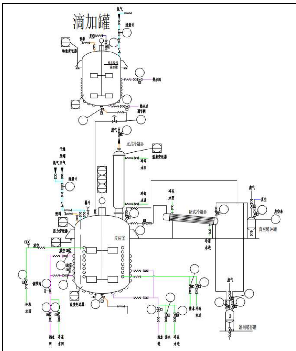
图4.3-10 UV固化阳离子有机硅树脂生产设备连接示意图
