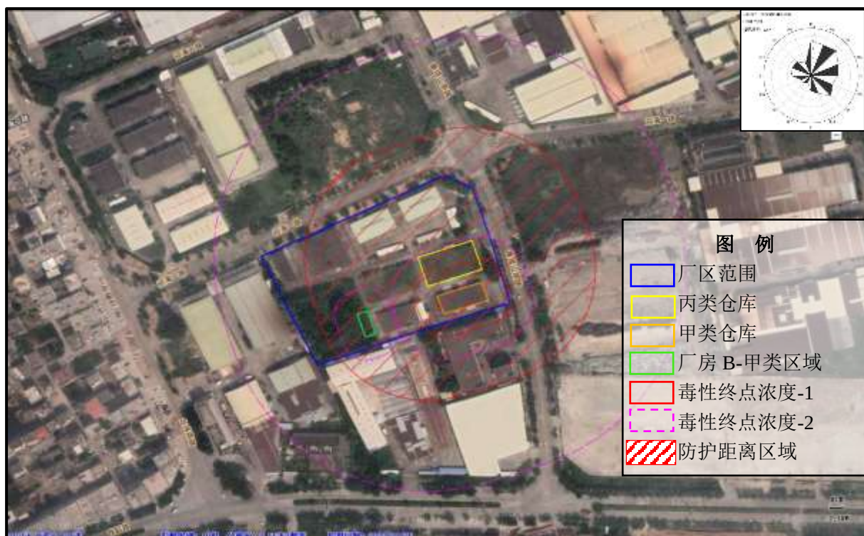
图9.5-1 本项目安全防护距离示意图
