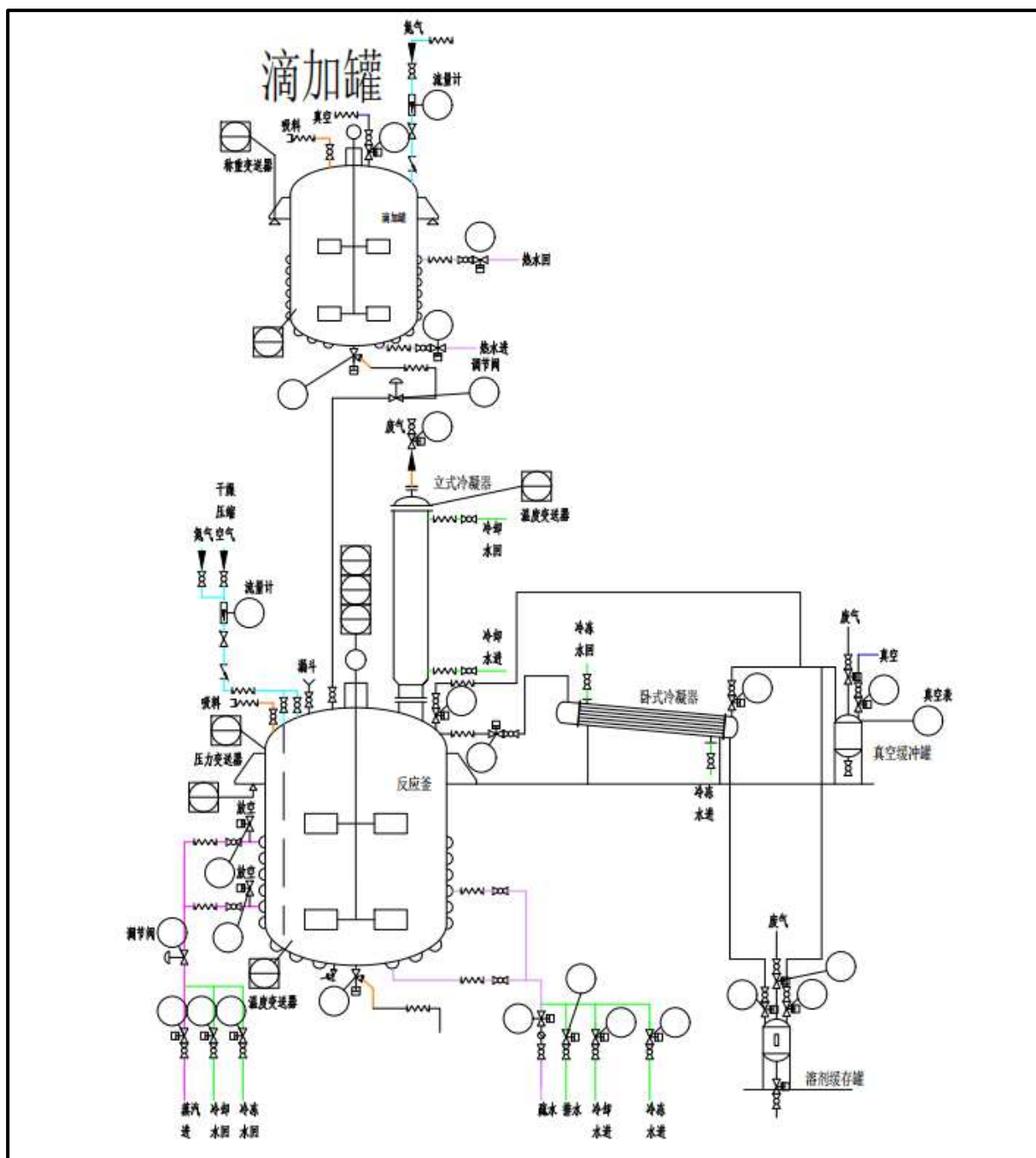
图4.3-4 聚氨酯丙烯酸酯树脂中间体生产设备连接示意图
