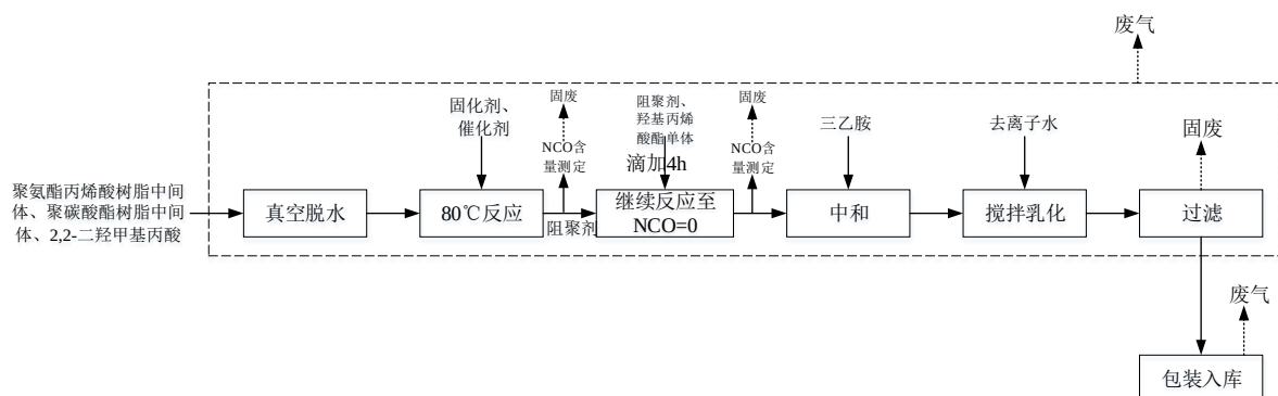
图 4.3-25 水性聚氨酯丙烯酸酯树脂乳液（本体法）工艺流程及产污环节
