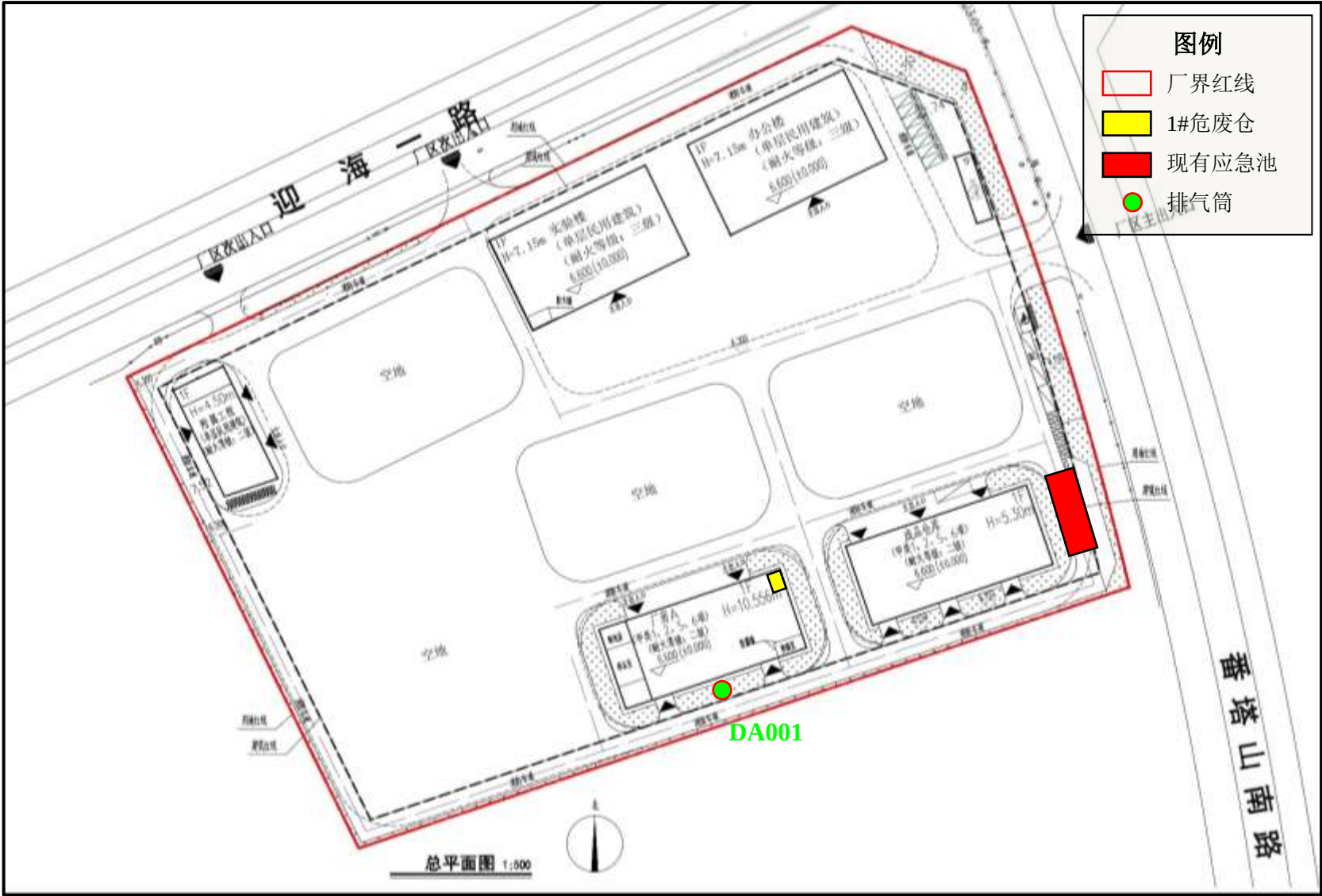
图3.5-1 现有项目平面布置图
