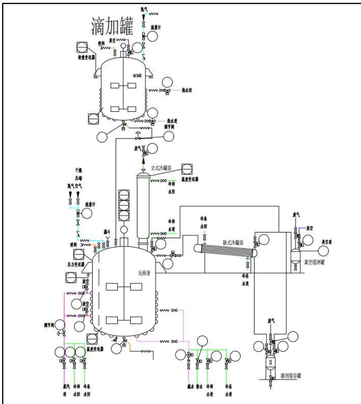
图4.3-32 有机硅改性聚氨酯丙烯酸酯树脂生产设备连接示意图
