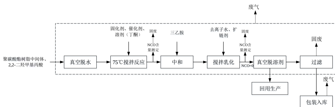
图 4.3-14 水性聚氨酯树脂乳液（溶液聚合法）工艺流程及产污环节
