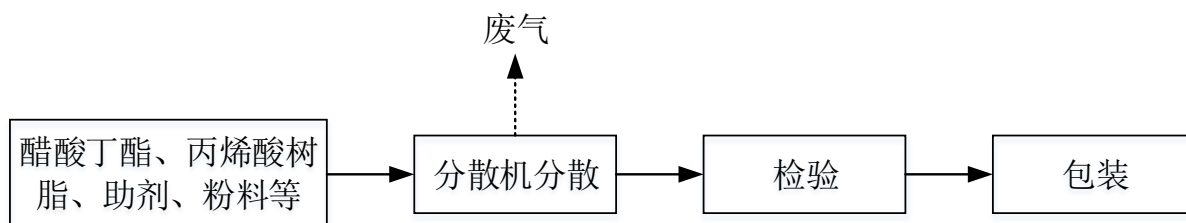
图 3.1-3 溶剂型丙烯酸树脂生产工艺流程
