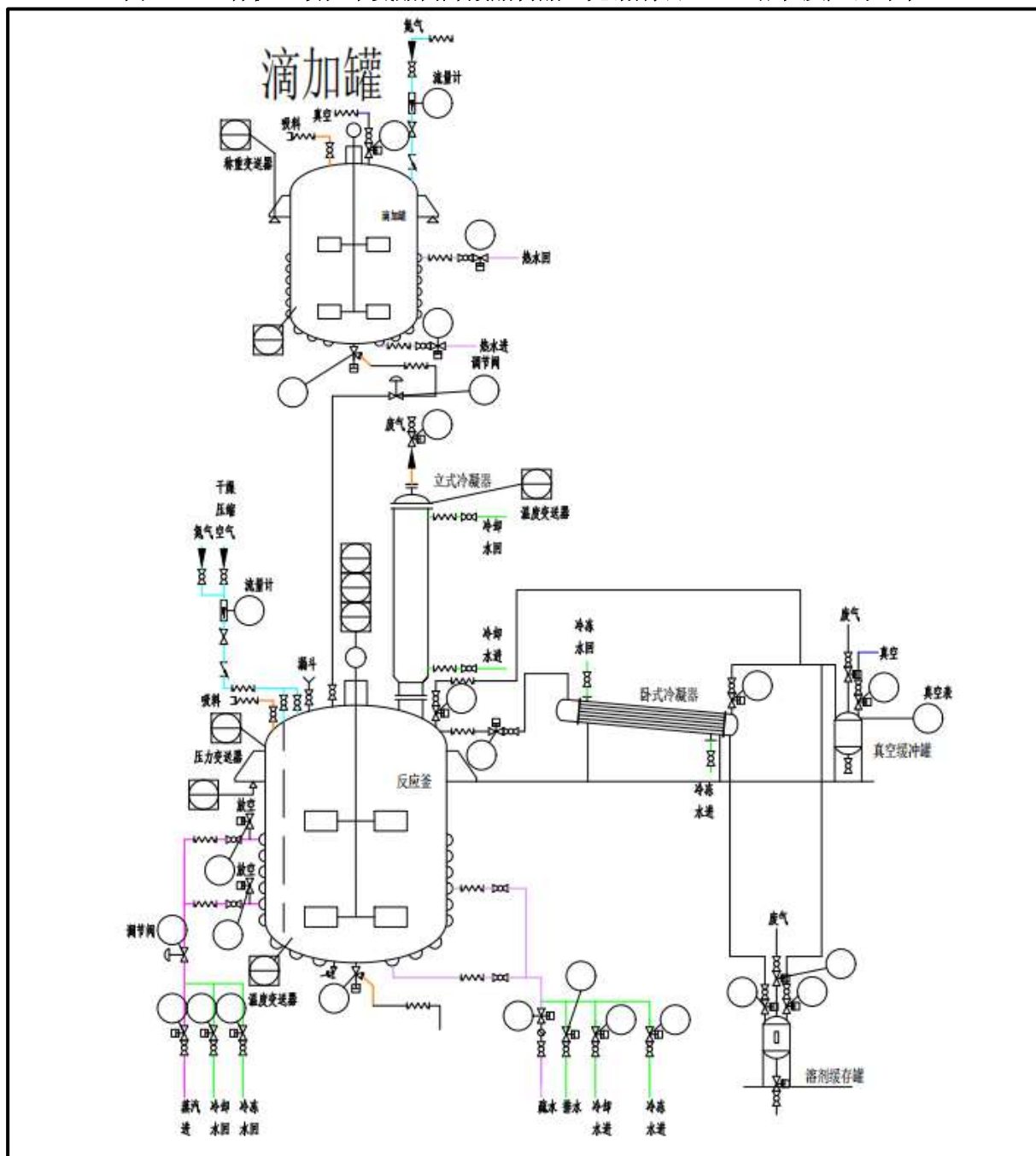
图 4.3-22 有机硅改性聚氨酯丙烯酸酯树脂生产设备连接示意图
