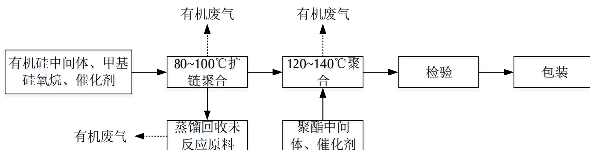
图 3.1-2 有机硅改性聚氨酯树脂生产工艺流程
