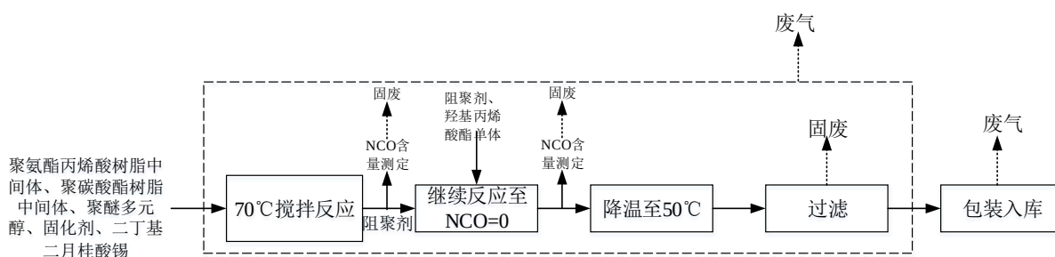
图 4.3-23 聚氨酯丙烯酸酯树脂（本体法，无溶剂）工艺流程及产污环节
