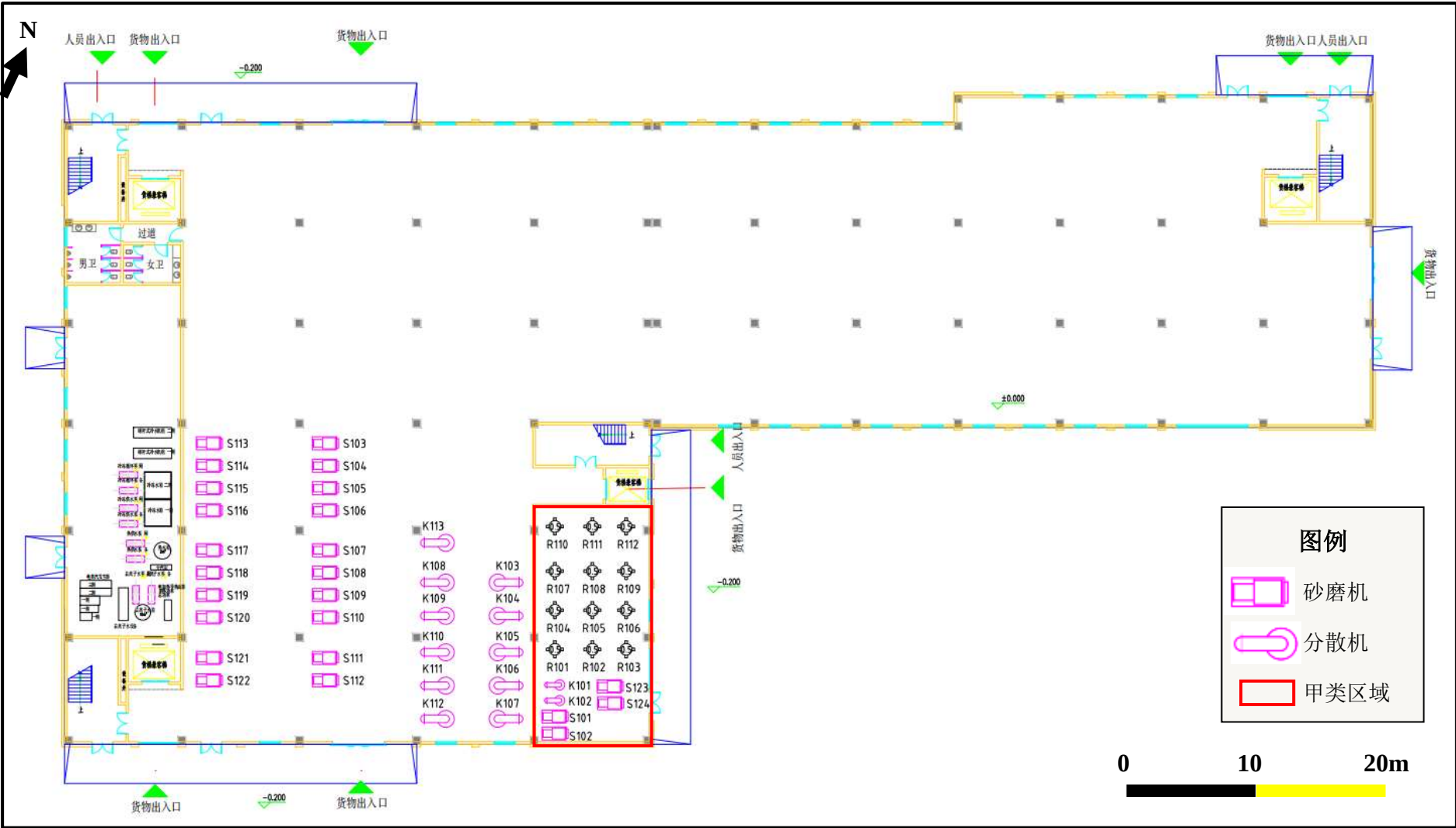
图3.5-3 厂房B车间平面布置图（1层）
