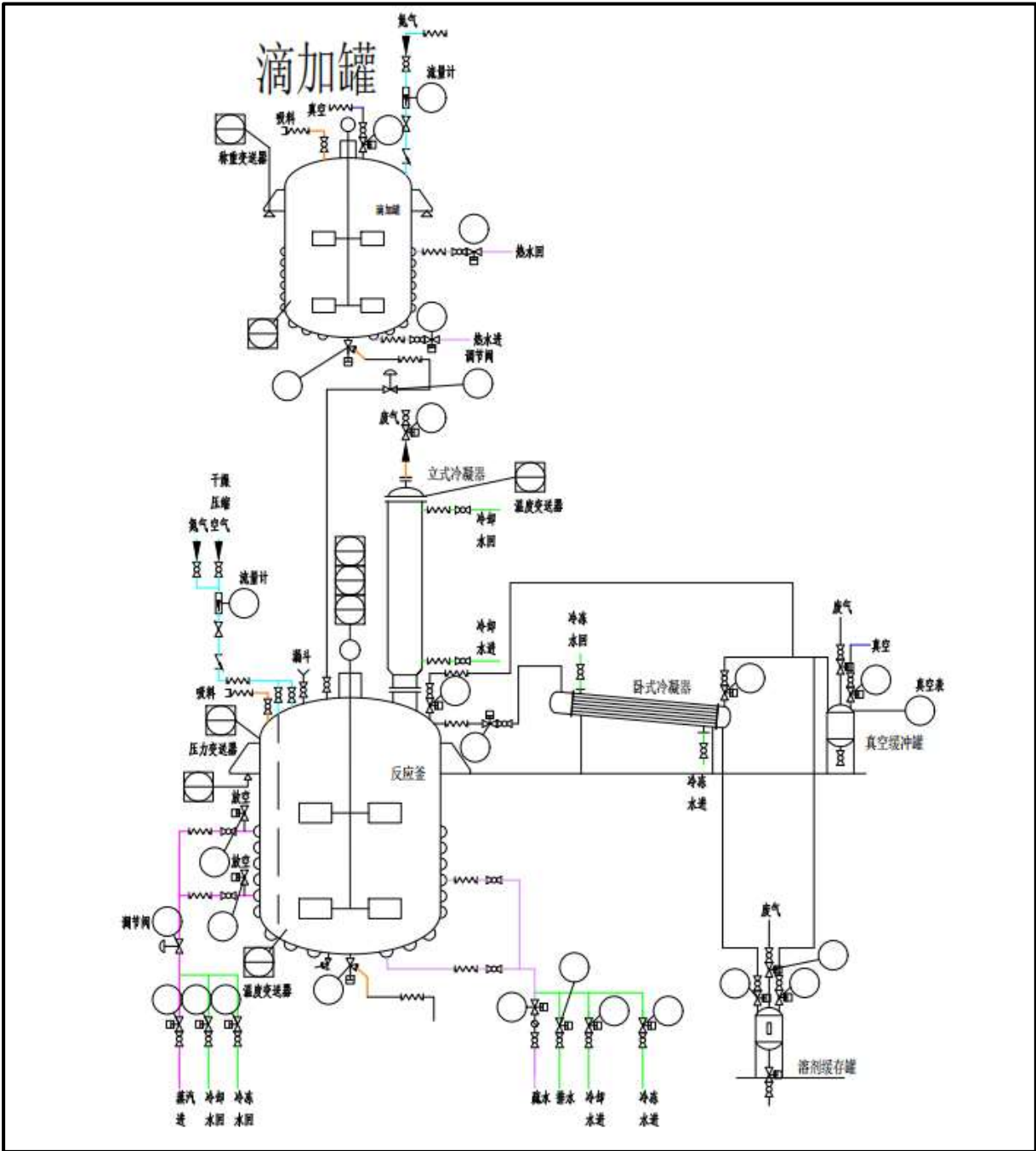
图4.3-24 聚氨酯丙烯酸酯树脂生产设备连接示意图
