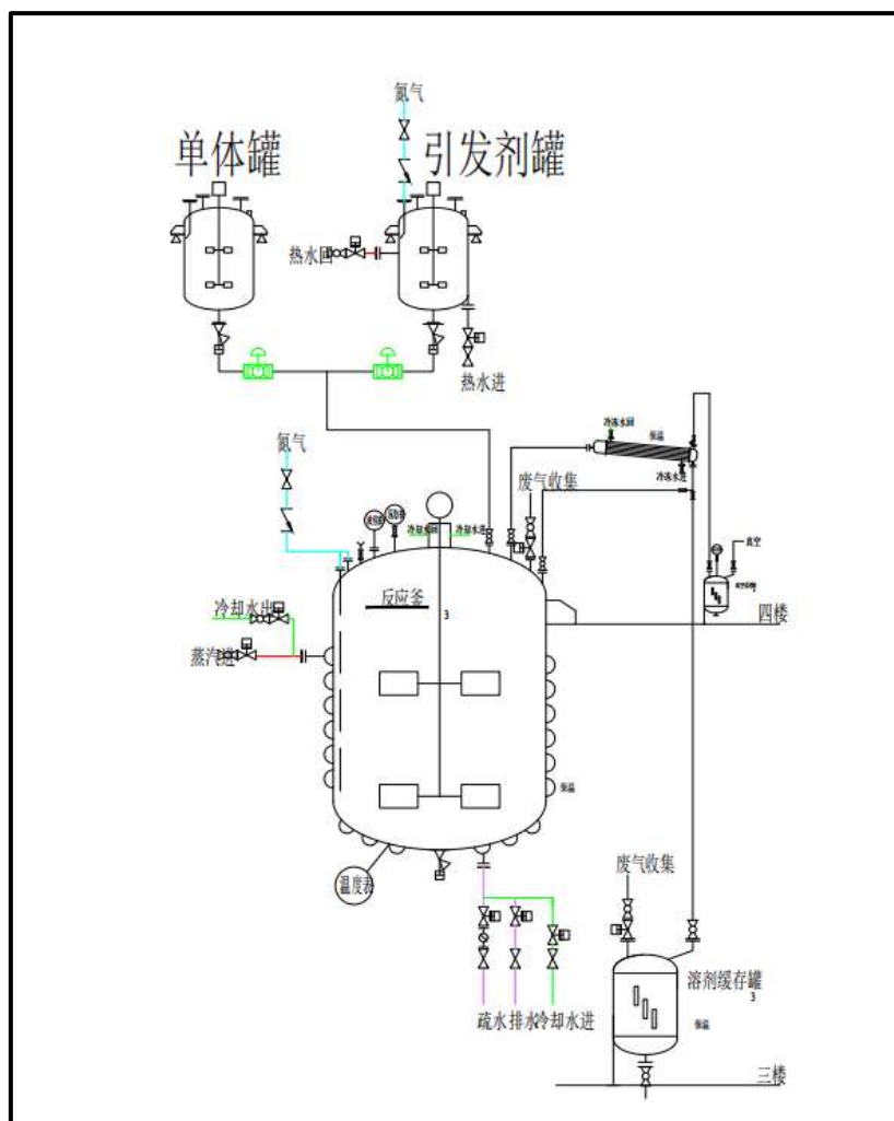
图4.3-2 丙烯酸树脂中间体生产设备连接示意图
