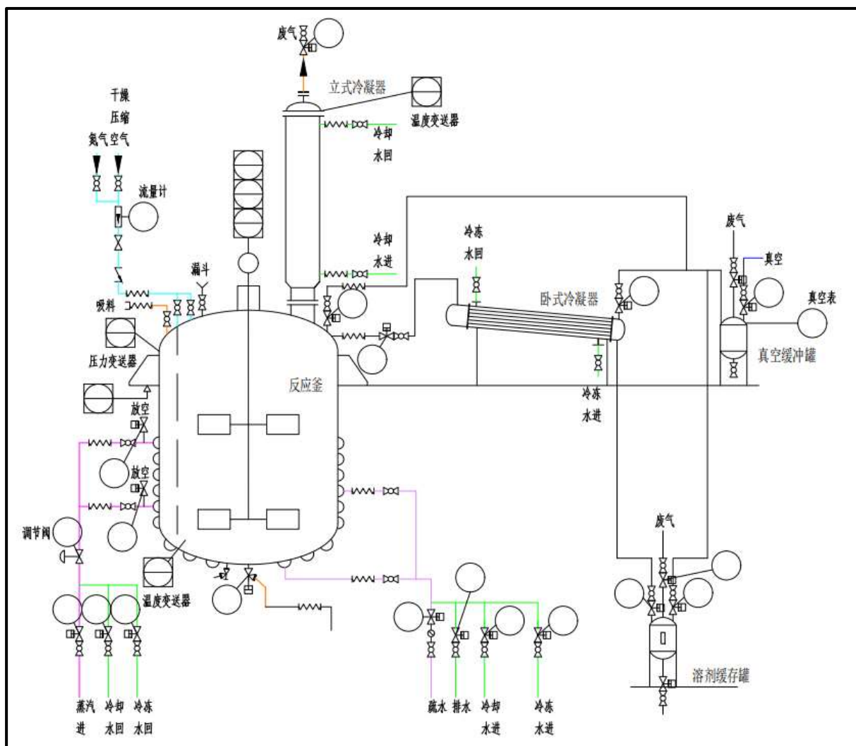
图4.3-8 纳米改性树脂中间体生产设备连接示意图
