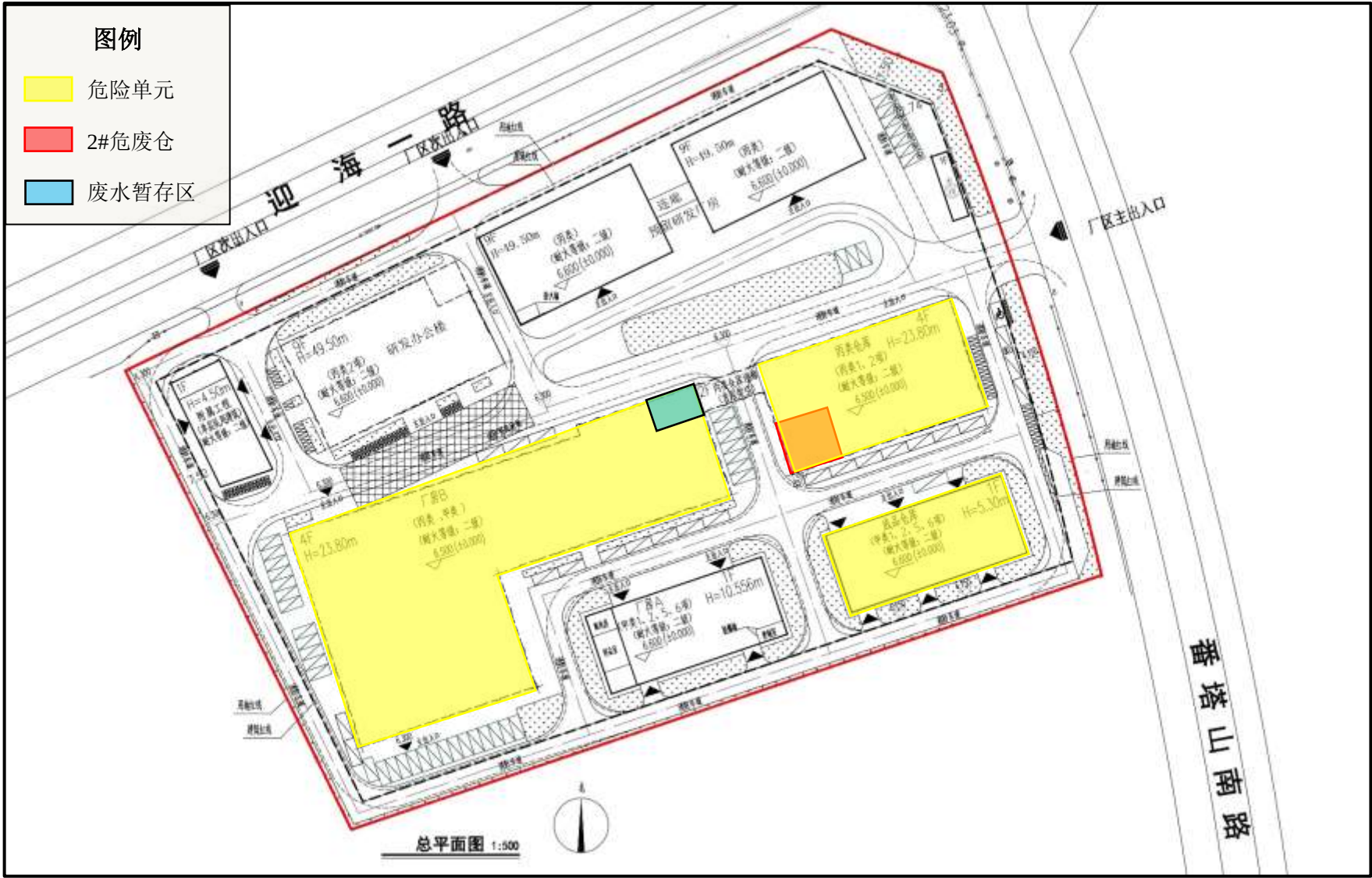
图9.3-1 本项目危险单元分布图
