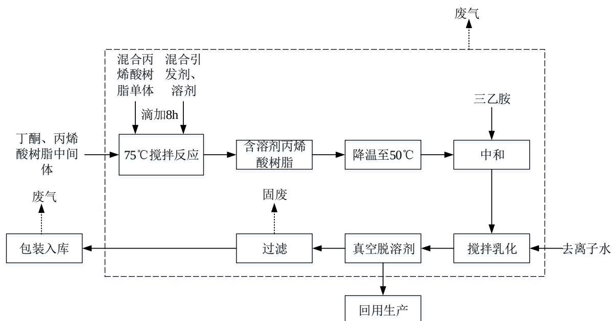
图 4.3-11 水性丙烯酸树脂乳液（溶液聚合法）工艺流程及产污环节
