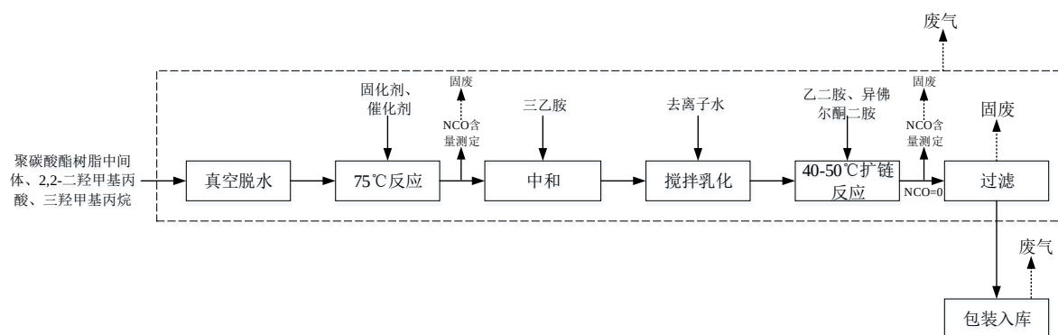
图 4.3-27 水性聚氨酯树脂乳液（无溶剂法）工艺流程及产污环节
