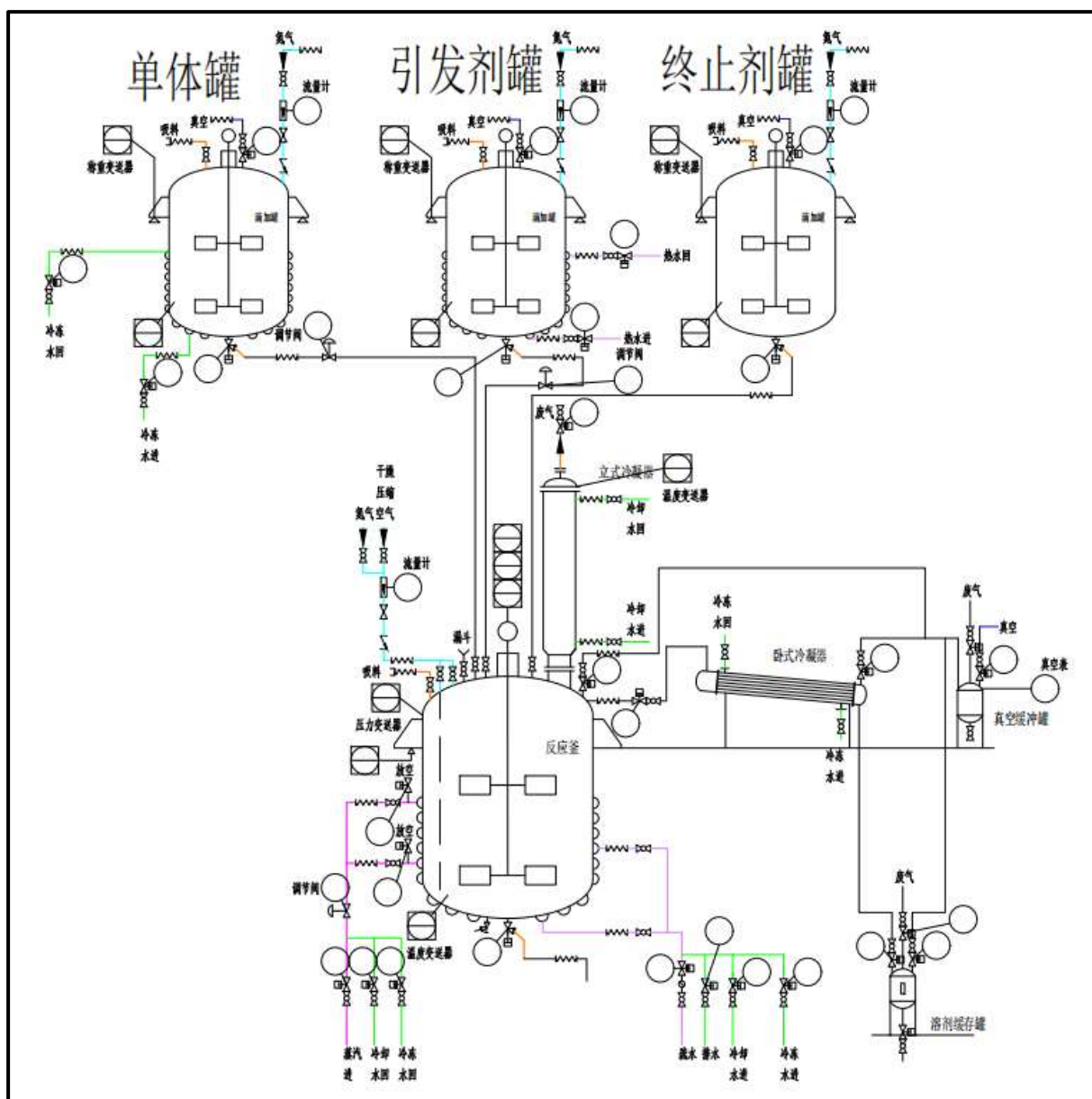
图4.3-12 水性丙烯酸树脂乳液生产设备连接示意图
