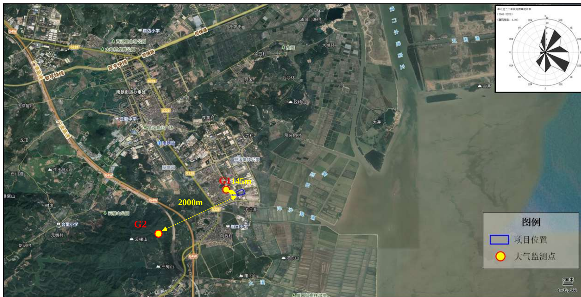
图6.1-3 大气监测布点
