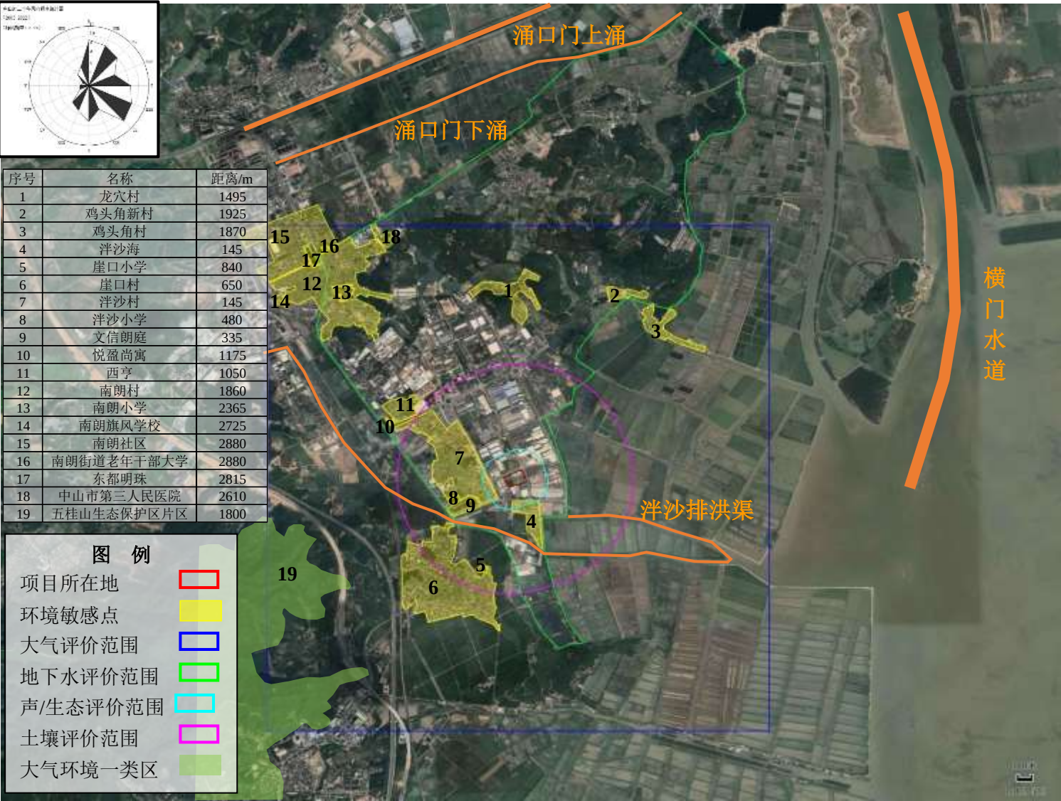
图 2.8-1 项目周边环境保护目标及控制目标图
