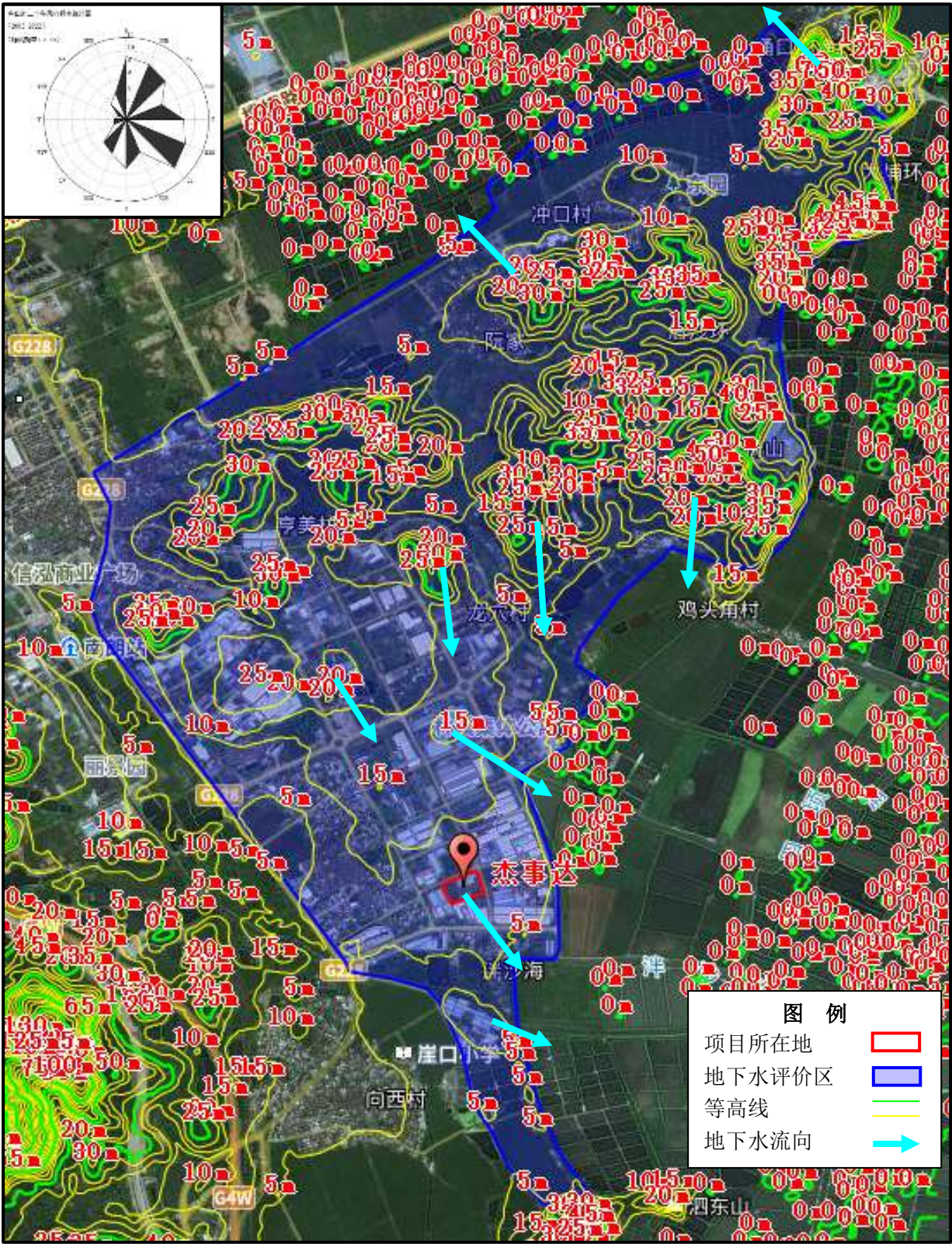
图7.3-5 地下水流向图
