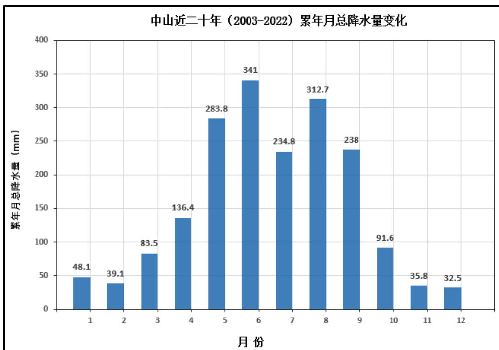
图7.4-6 中山基本站月平均降水量（单位：毫米）
