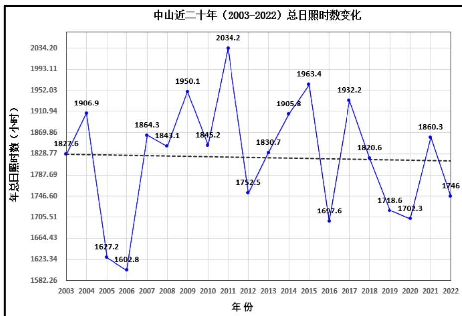
图7.4-9 中山基本站年日照时长（单位：小时，虚线为趋势线）
