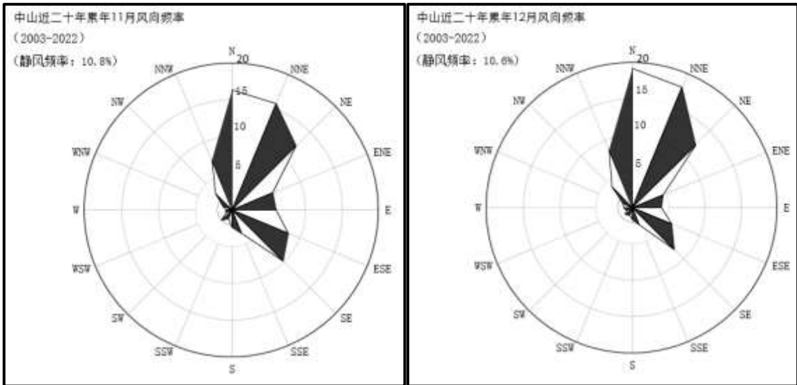
图7.4-2 中山基本站月风向玫瑰图
