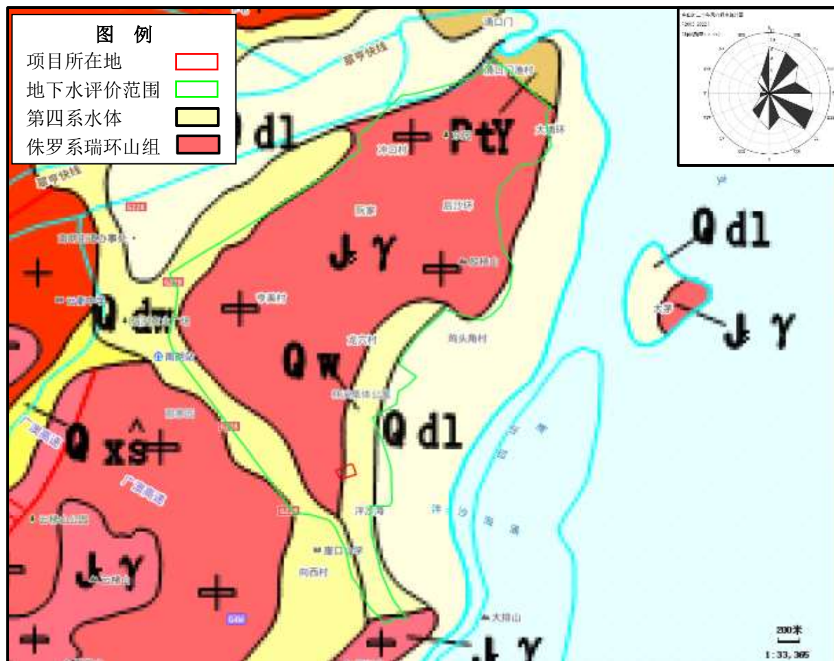
图2.6-2 地下水评价范围图（地质图）
