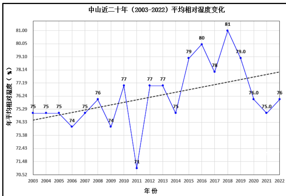
图7.4-11 中山基本站年平均相对湿度（纵轴为百分比，虚线为趋势线）
