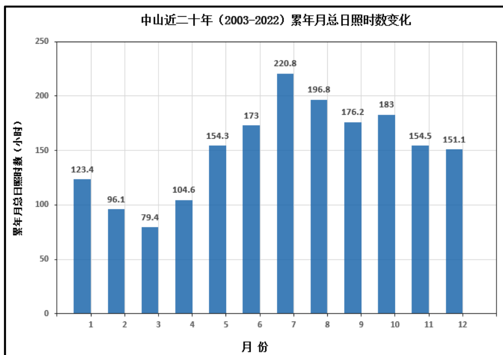
图7.4-8 中山基本站月日照时数（单位：小时）
