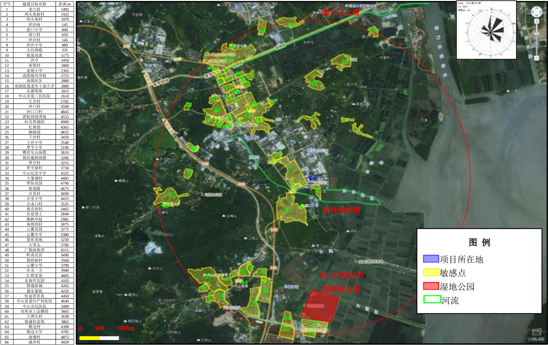
图9.2-2 环境风险敏感目标图
