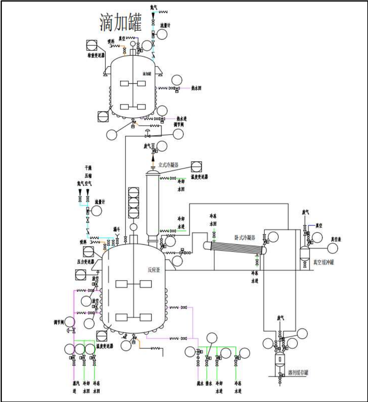
图4.3-6 有机硅树脂中间体生产设备连接示意图
