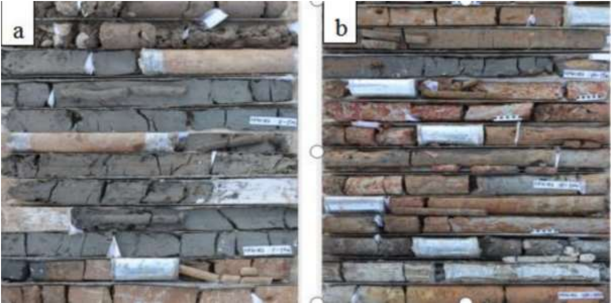
图7.3-1 钻孔岩芯照片
