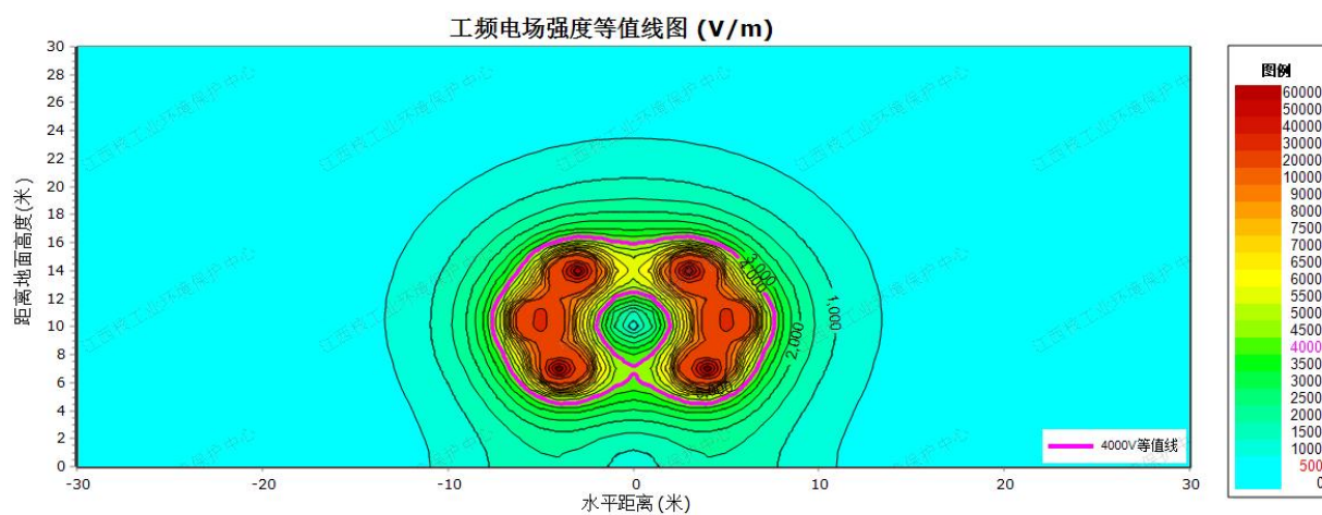
图 4-8 输电线路理论计算工频电场强度等值线图
