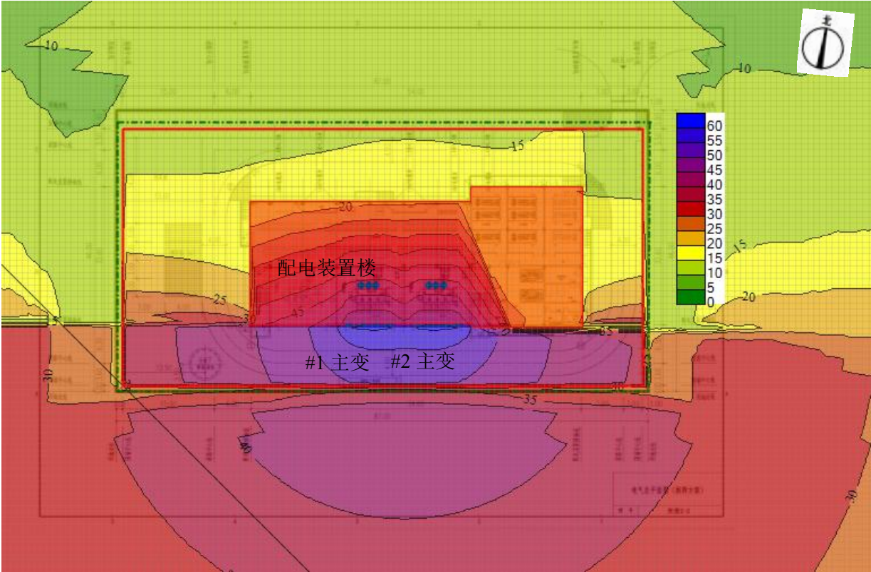
图 4-4 110 千伏外沙站噪声等声级线图
