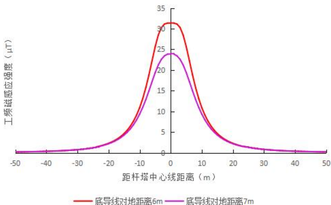
图 4-9 输电线路理论计算工频磁感应强度曲线图
