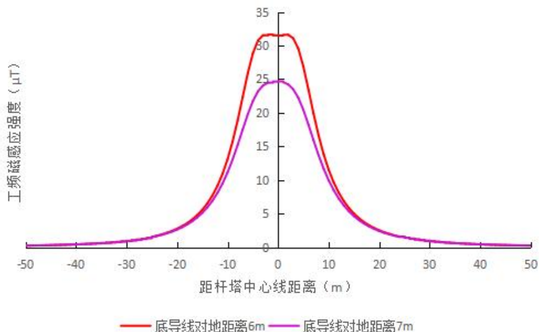
图 4-5 输电线路理论计算工频磁感应强度曲线图
