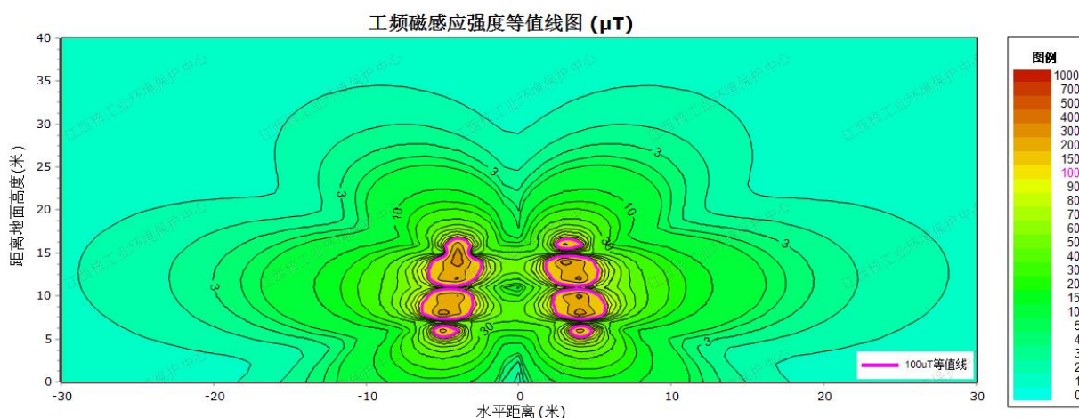
图 4-6 输电线路理论计算工频磁感应强度等值线图
