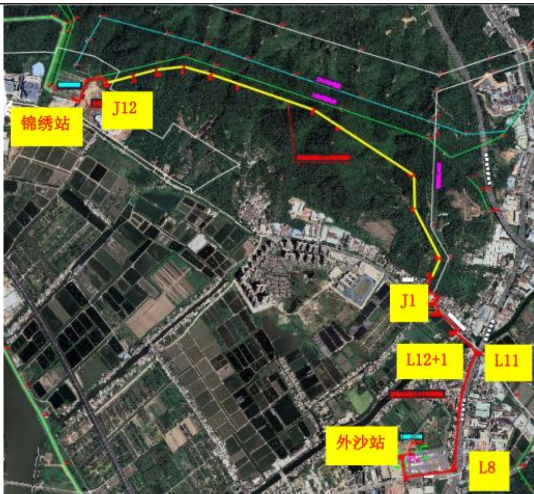
图 2-2 110kV 锦绣至外沙线路工程路径示意图
