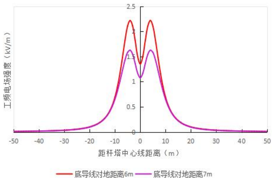
图 4-7 输电线路理论计算工频电场强度曲线图
