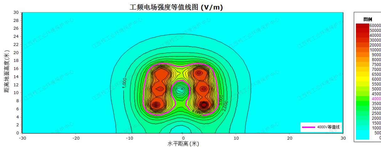
图 4-4 输电线路理论计算工频电场强度等值线图
