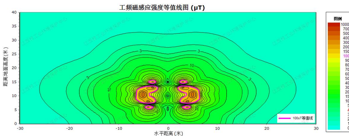
图 4-10 输电线路理论计算工频磁感应强度等值线图
