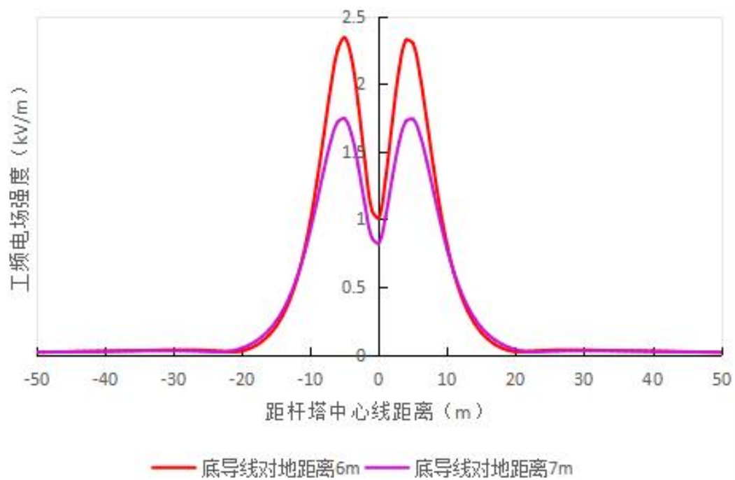
图 4-3 输电线路理论计算工频电场强度曲线图
