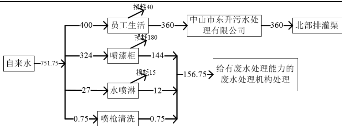
图 1 水平衡图
