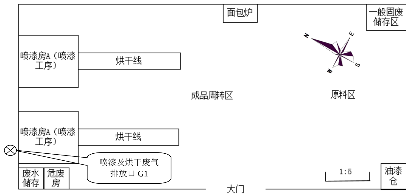
附图 3 建设项目平面布置图
