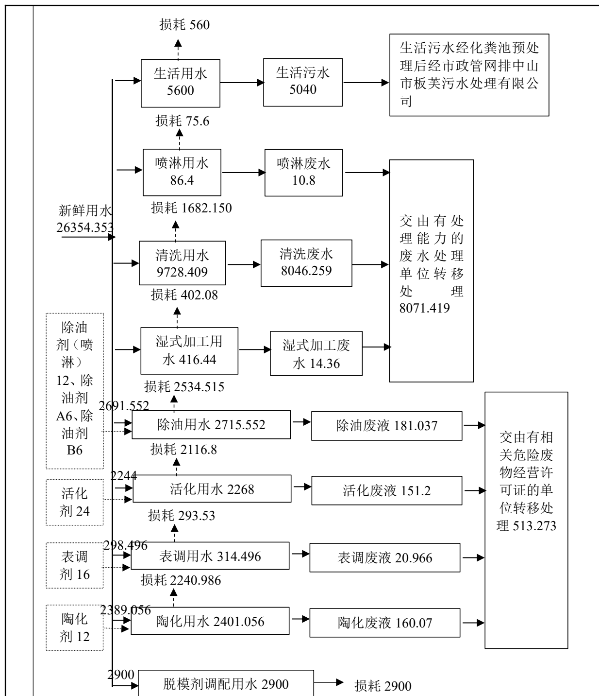
图3 改扩建后水平衡图 (单位: t/a)
