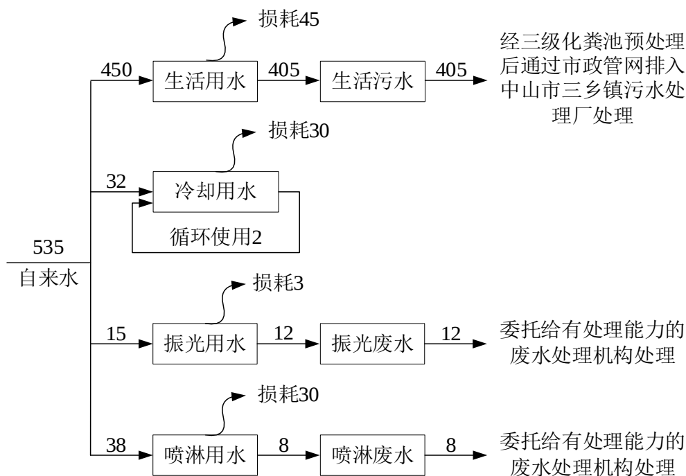
图1 项目水平衡图 (t/a)
