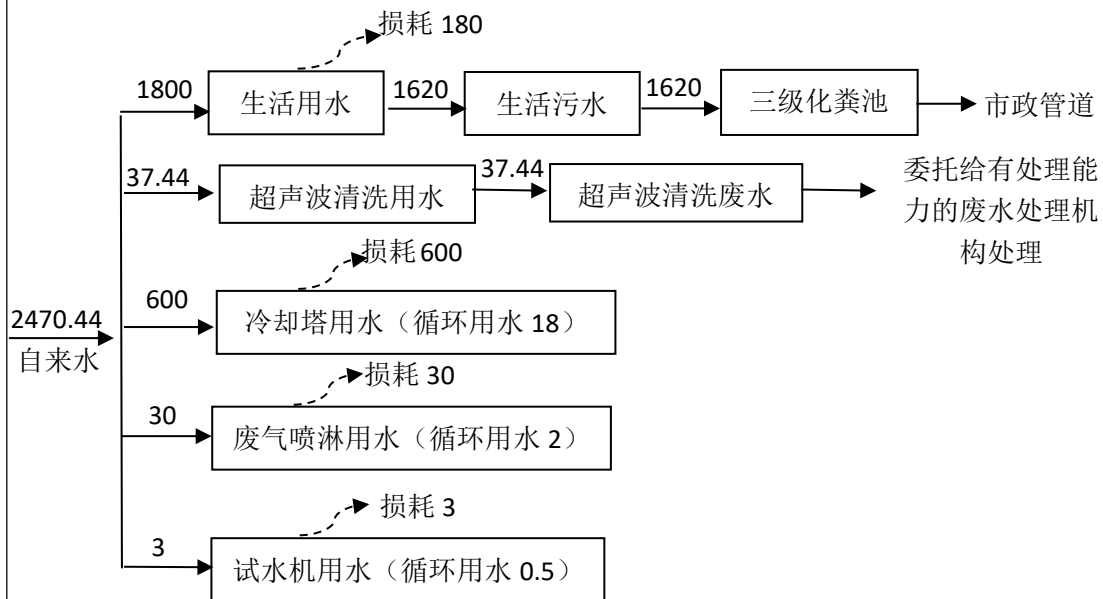
图 2-1 项目扩建前水量平衡图 (t/a)
