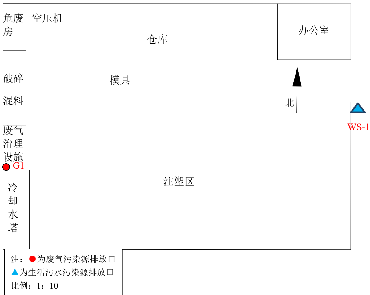
图 5 建设项目厂区总平面布置图
