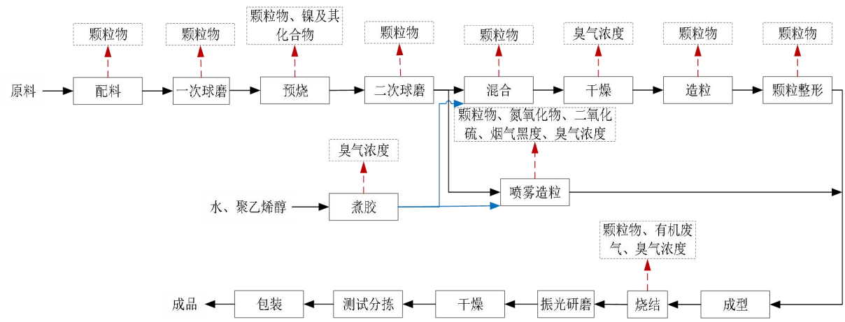
工艺流程图
