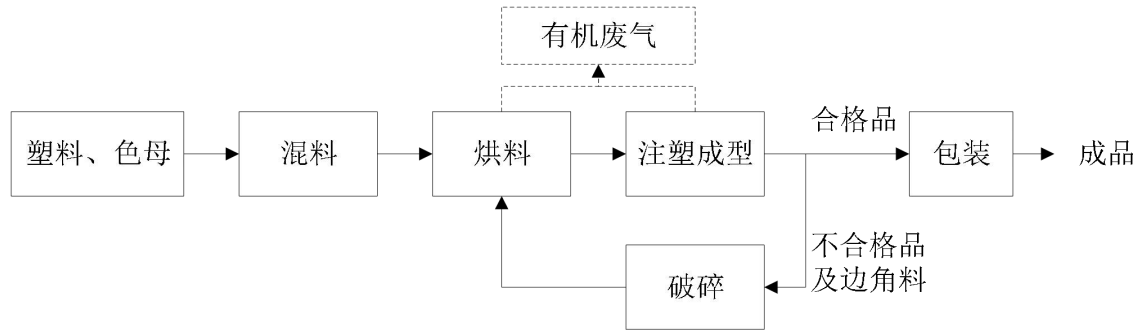
图 2 工艺流程图
