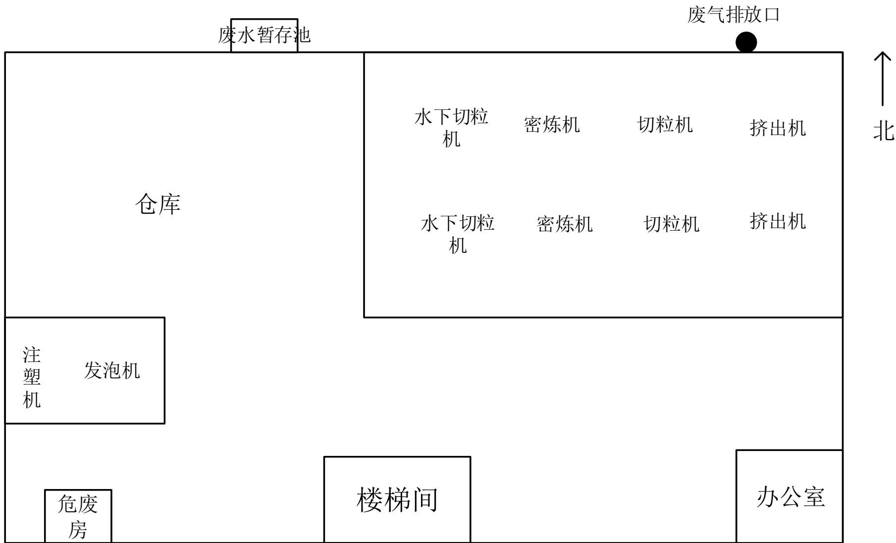
图三 建设项目 1 楼平面布置图
