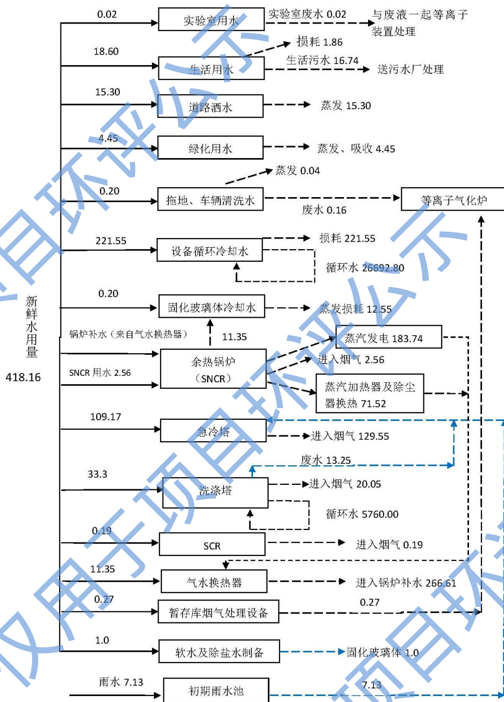
图1项目建成后全厂水平衡图 (单位: m³/d)
