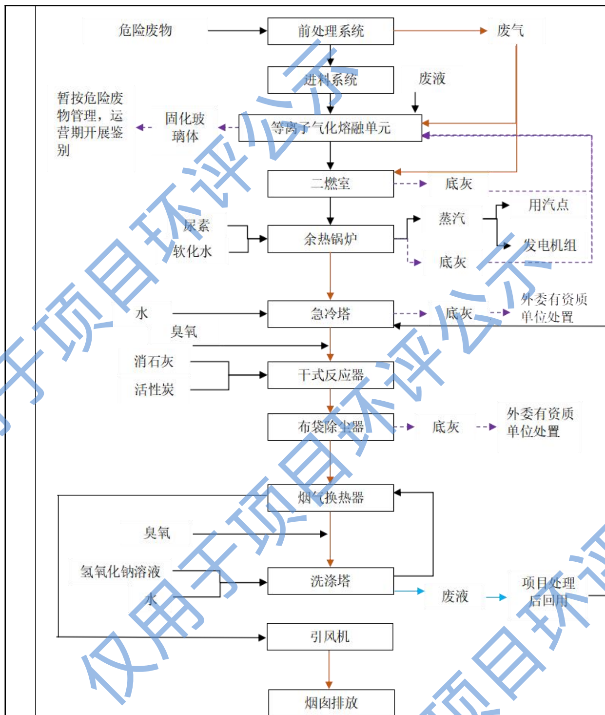
图3工艺流程及产污节点简图
