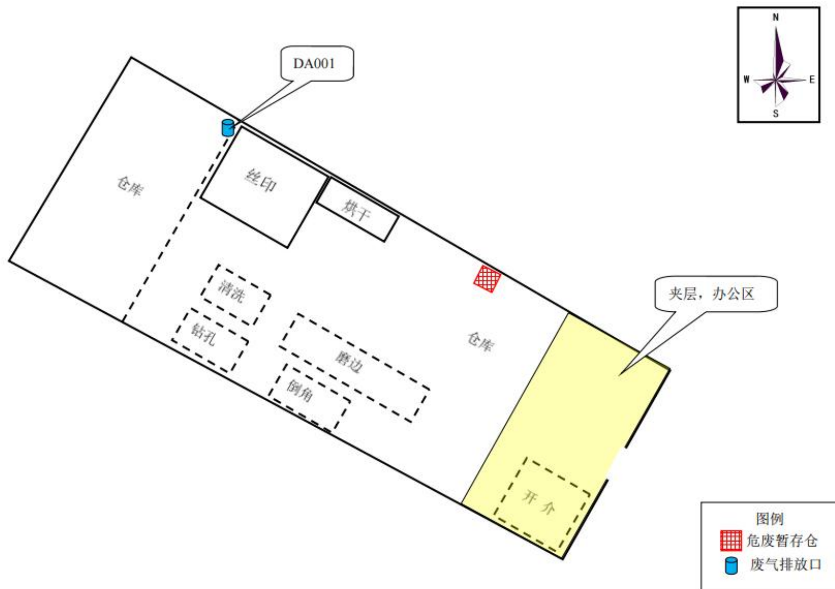
附图3 生产车间平面布置图
