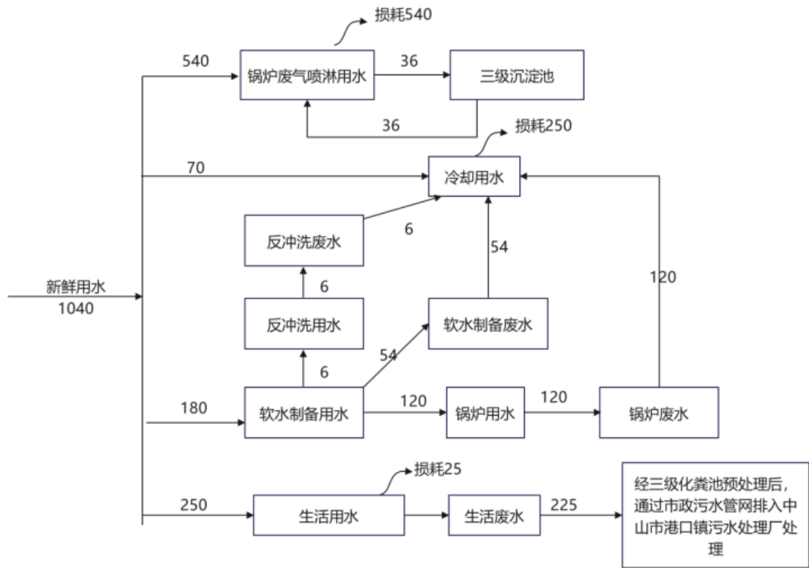
图 1 扩建前原有部分水平衡图 单位: \text{m}^3/\text{a}
