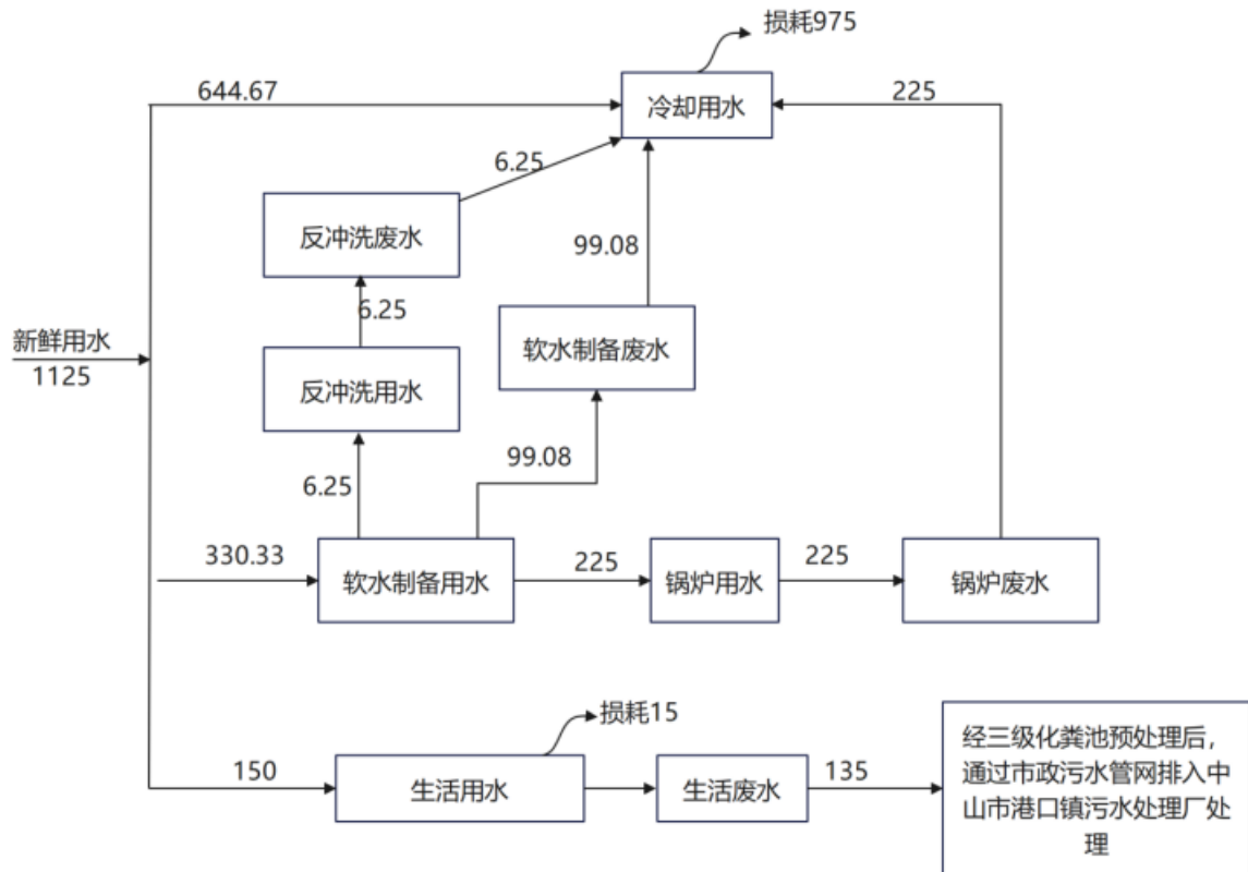
图 1 扩建后水平衡图 单位: m 3 /a
